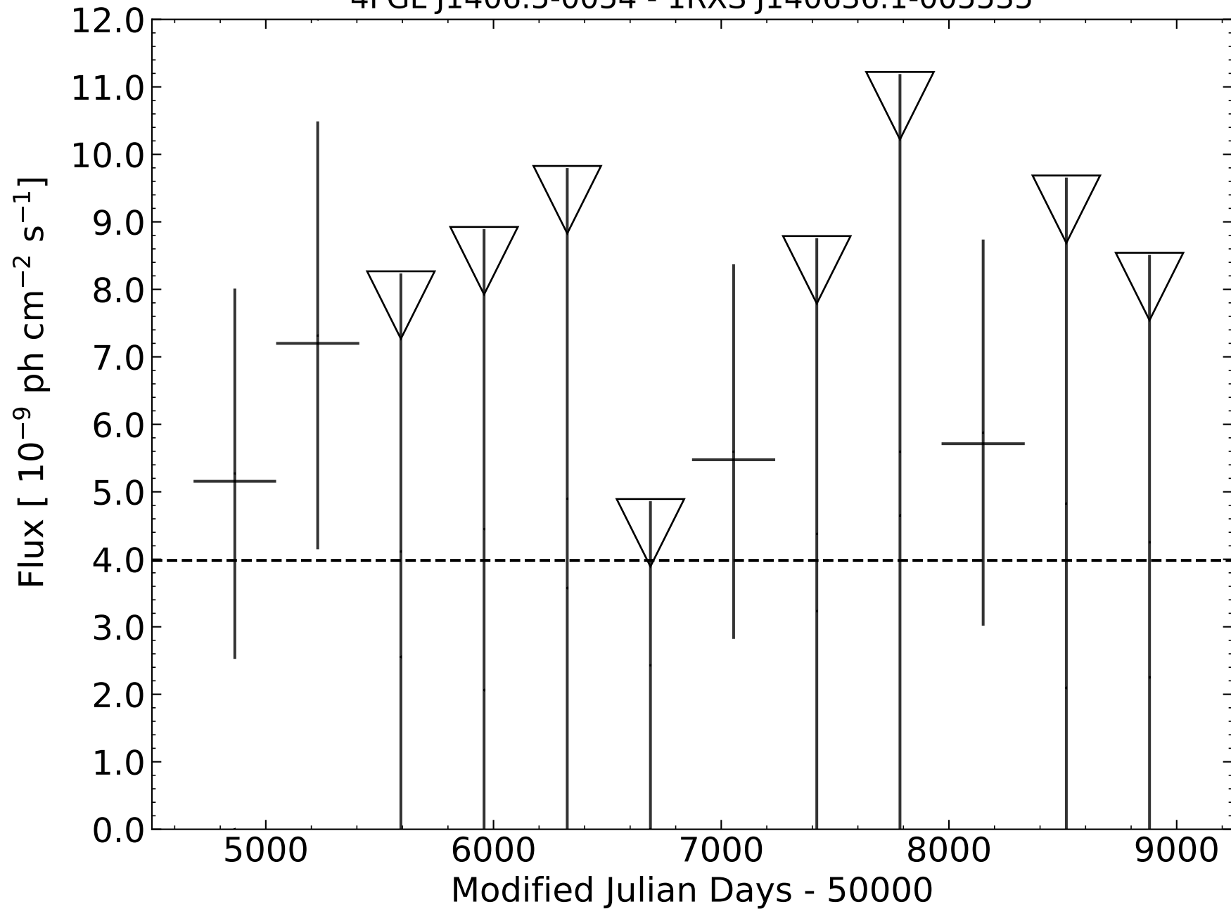
4FGL J1406.5-0054 - 1RXS J140636.1-005535
