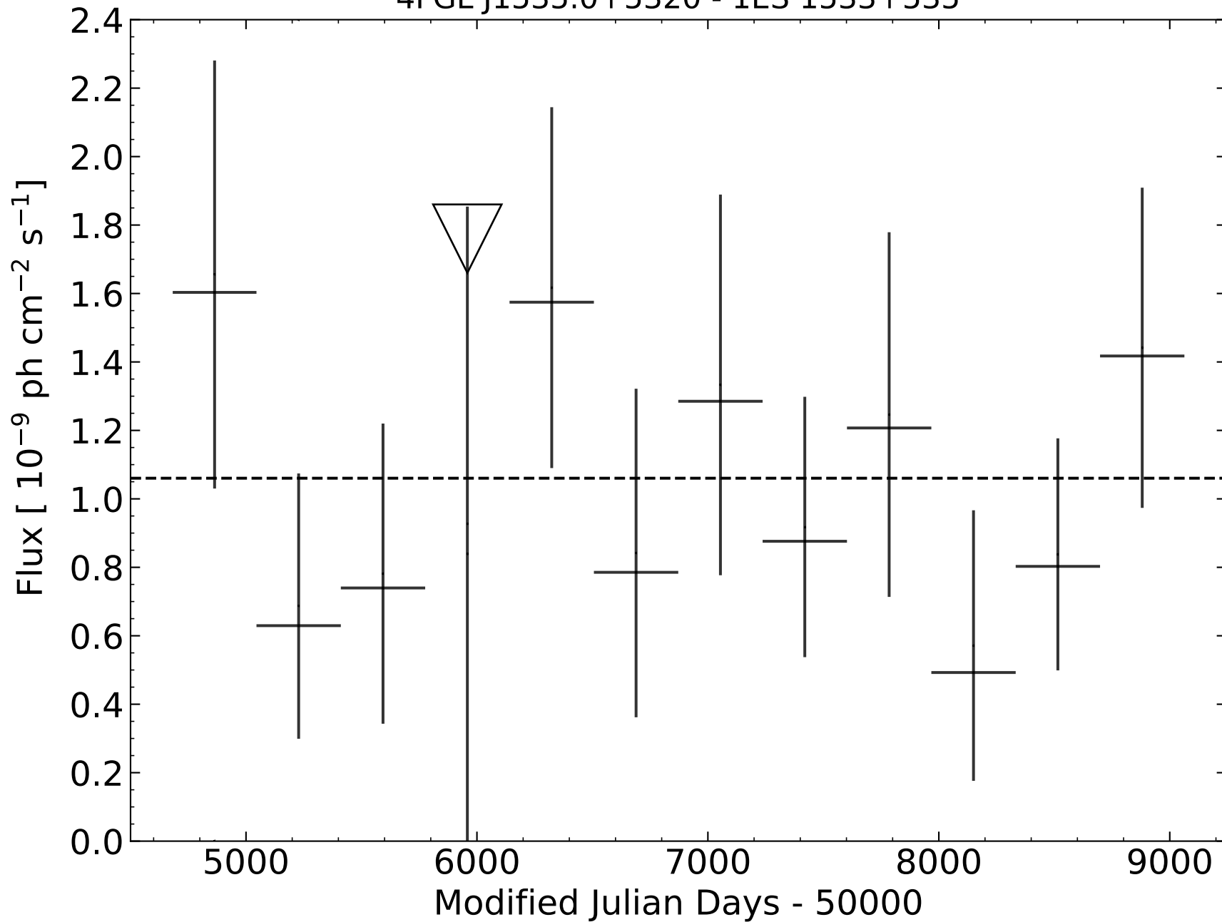
4FGL J1535.0+5320 - 1ES 1533+535
