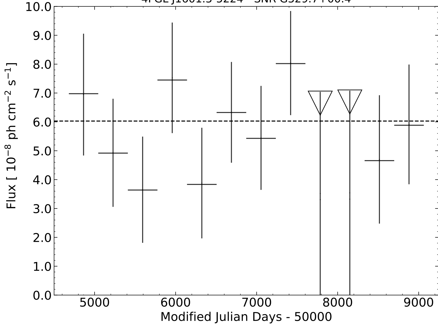
4FGL J1601.3-5224 - SNR G329.7+00.4
