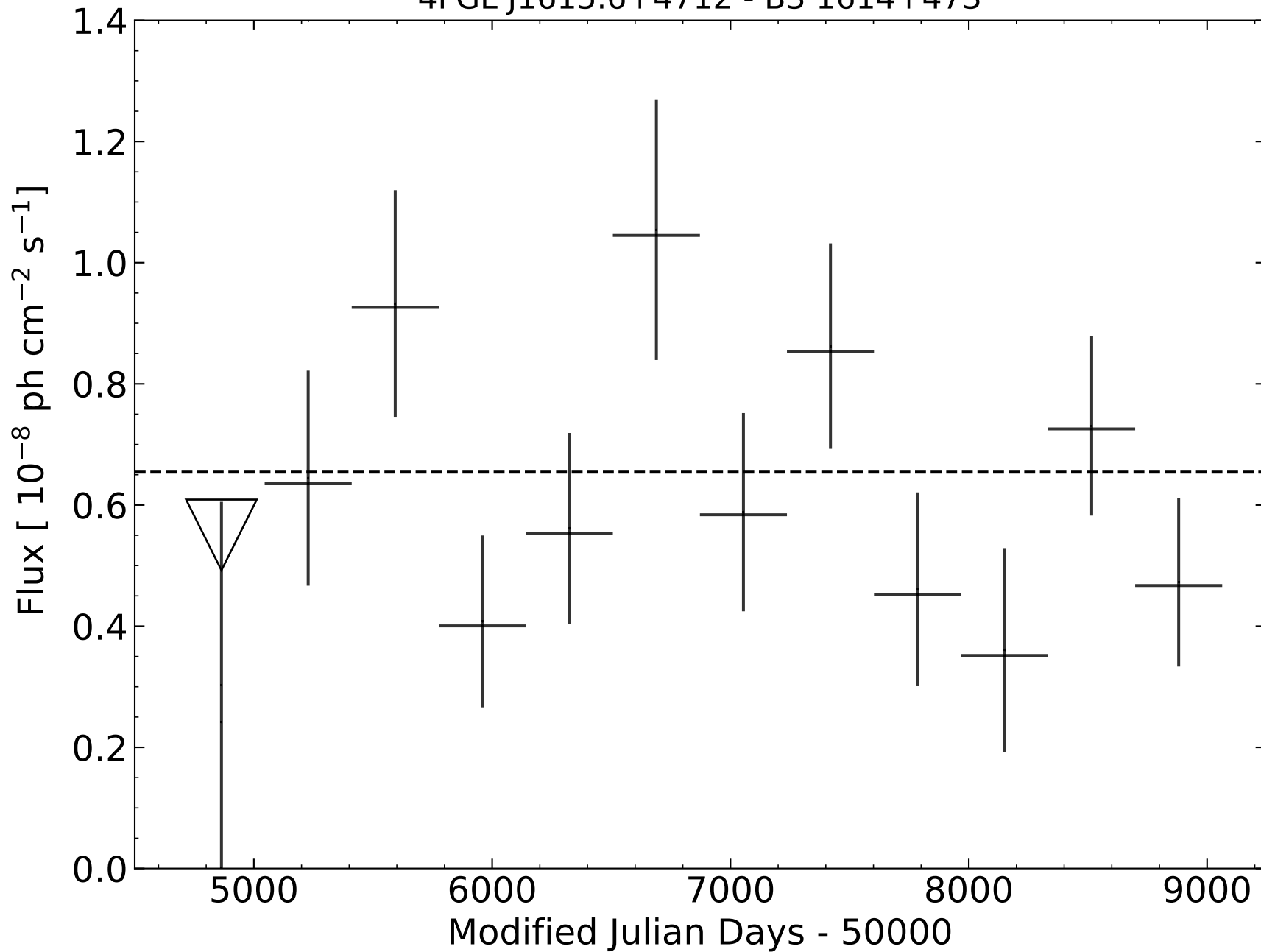
4FGL J1615.6+4712 - B3 1614+473
