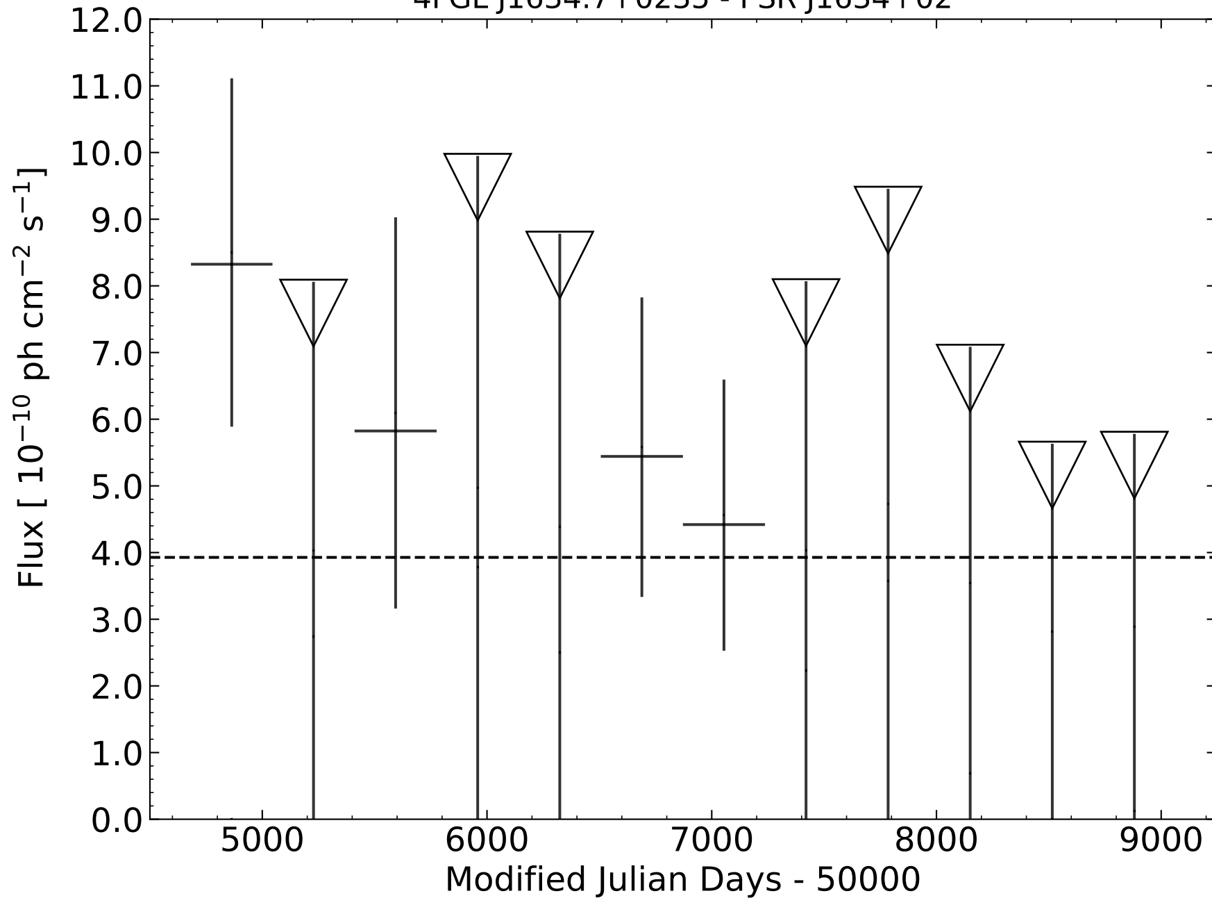
4FGL J1634.7+0235 - PSR J1634+02
