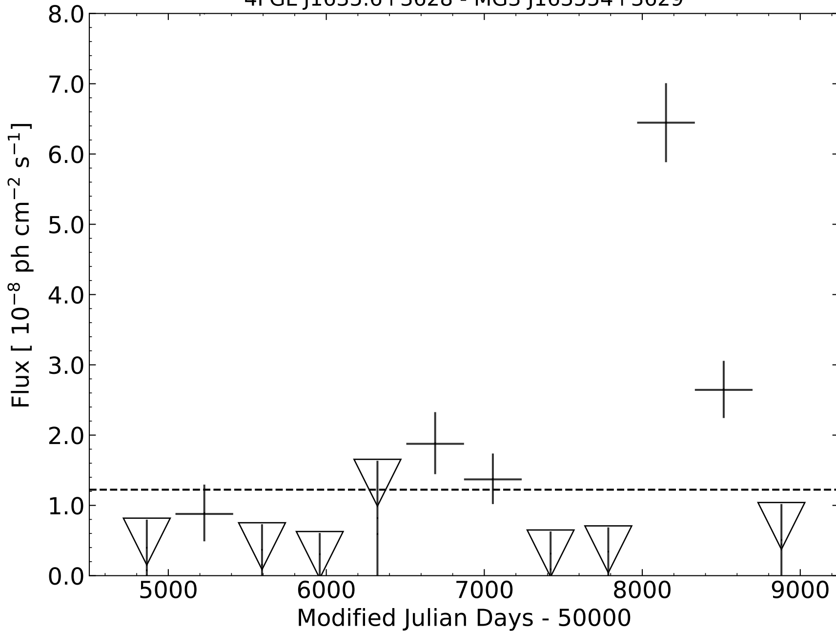
4FGL J1635.6+3628 - MG3 J163554+3629
