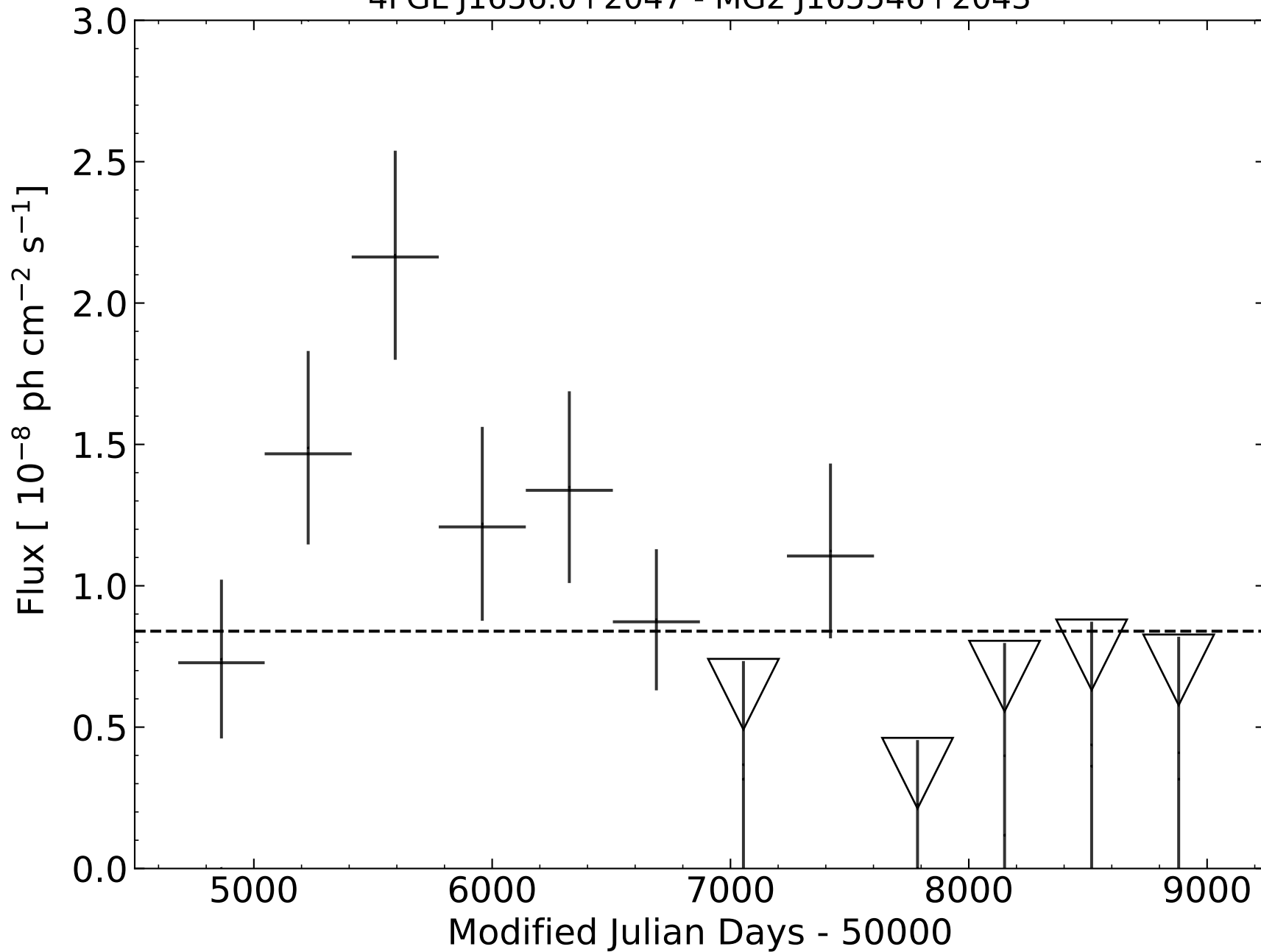
4FGL J1656.0+2047 - MG2 J165546+2043
