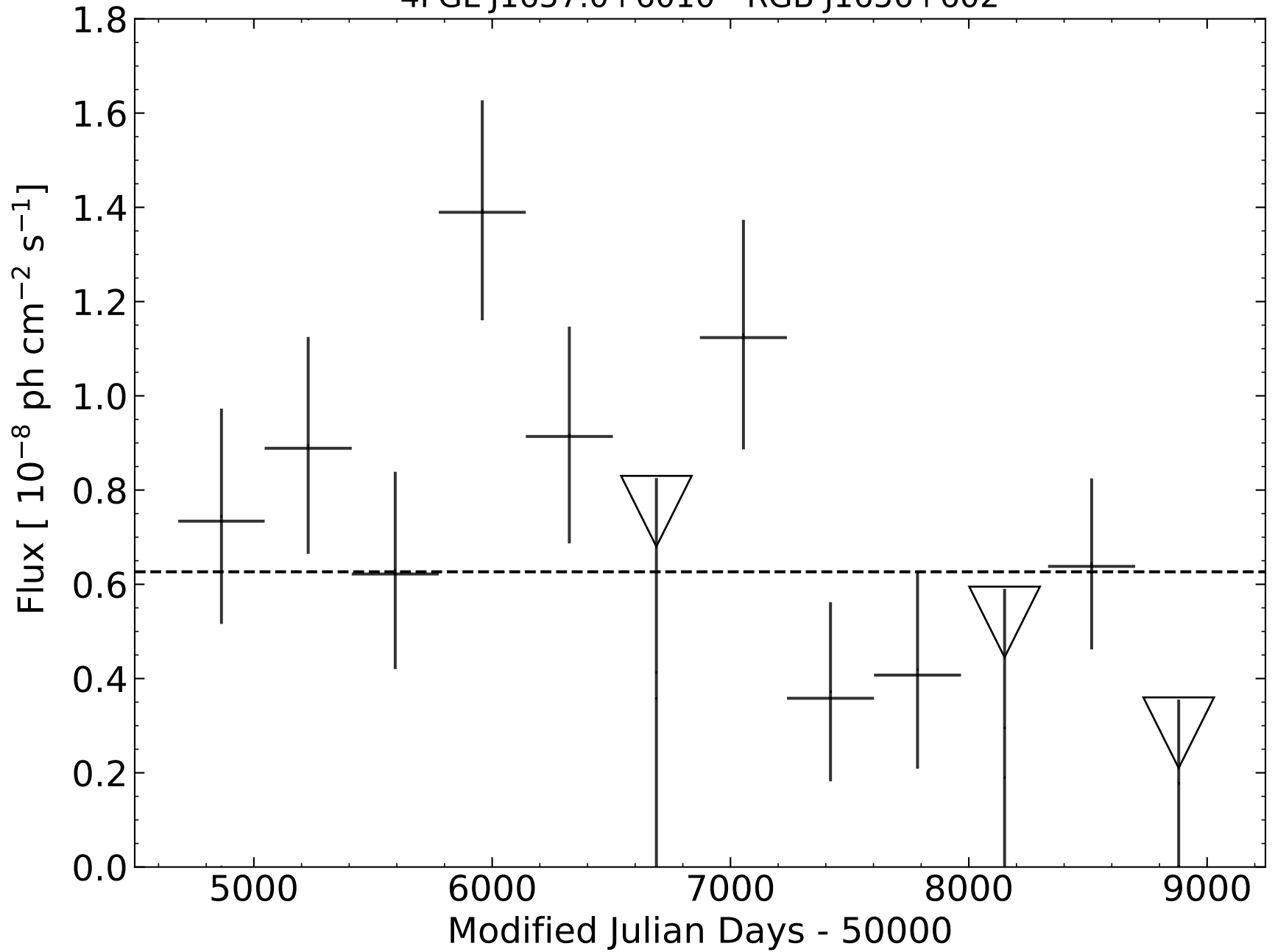
4FGL J1657.0+6010 - RGB J1656+602
