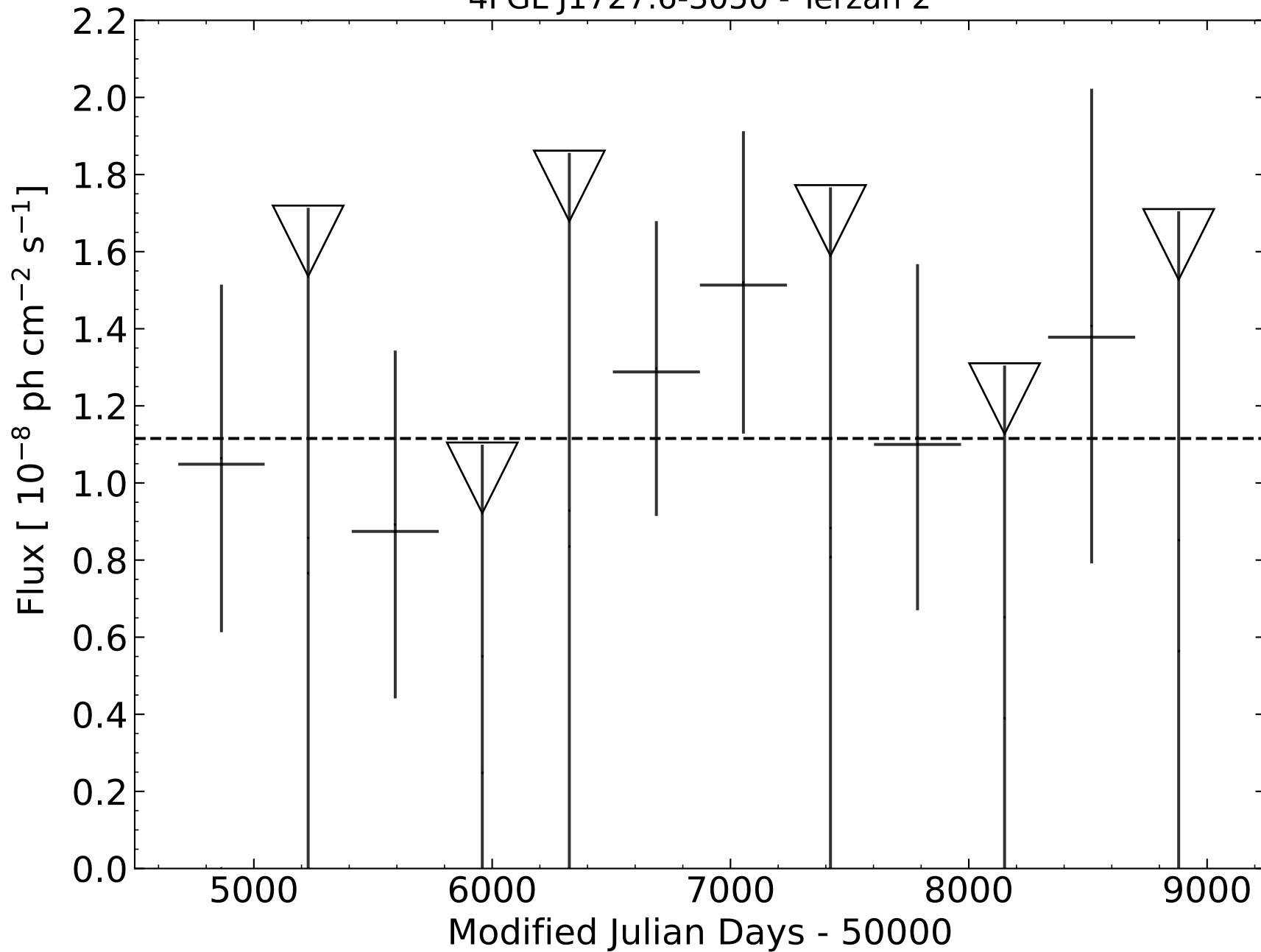
4FGL J1727.6-3050 - Terzan 2
