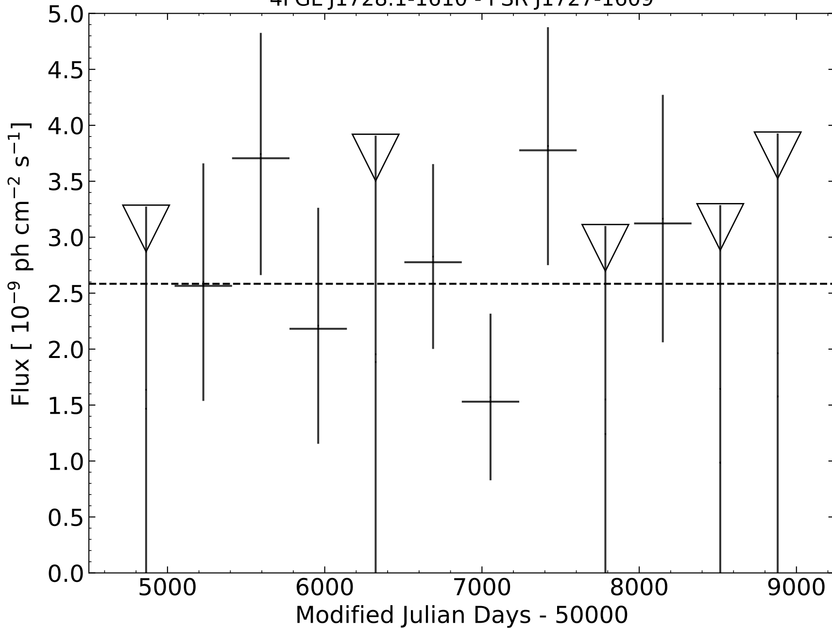
4FGL J1728.1-1610 - PSR J1727-1609
