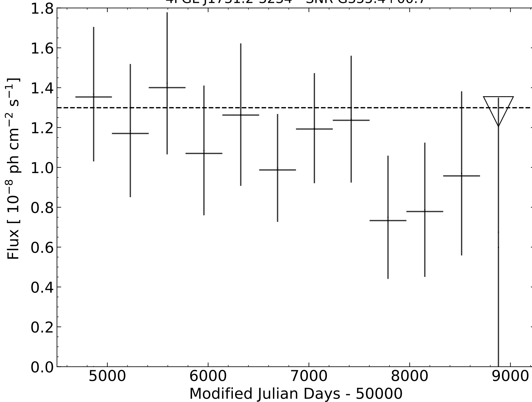
4FGL J1731.2-3234 - SNR G355.4+00.7
