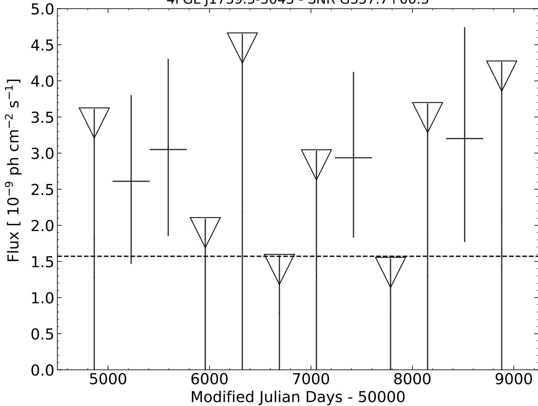
4FGL J1739.5-3043 - SNR G357.7+00.3
