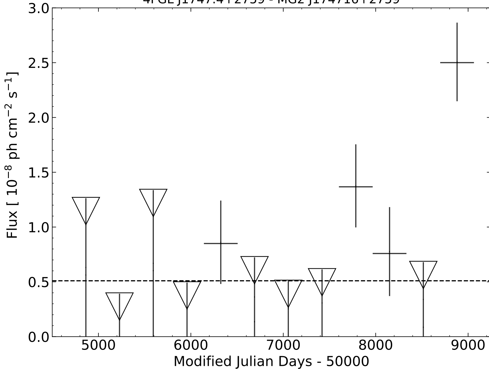
4FGL J1747.4+2759 - MG2 J174716+2759
