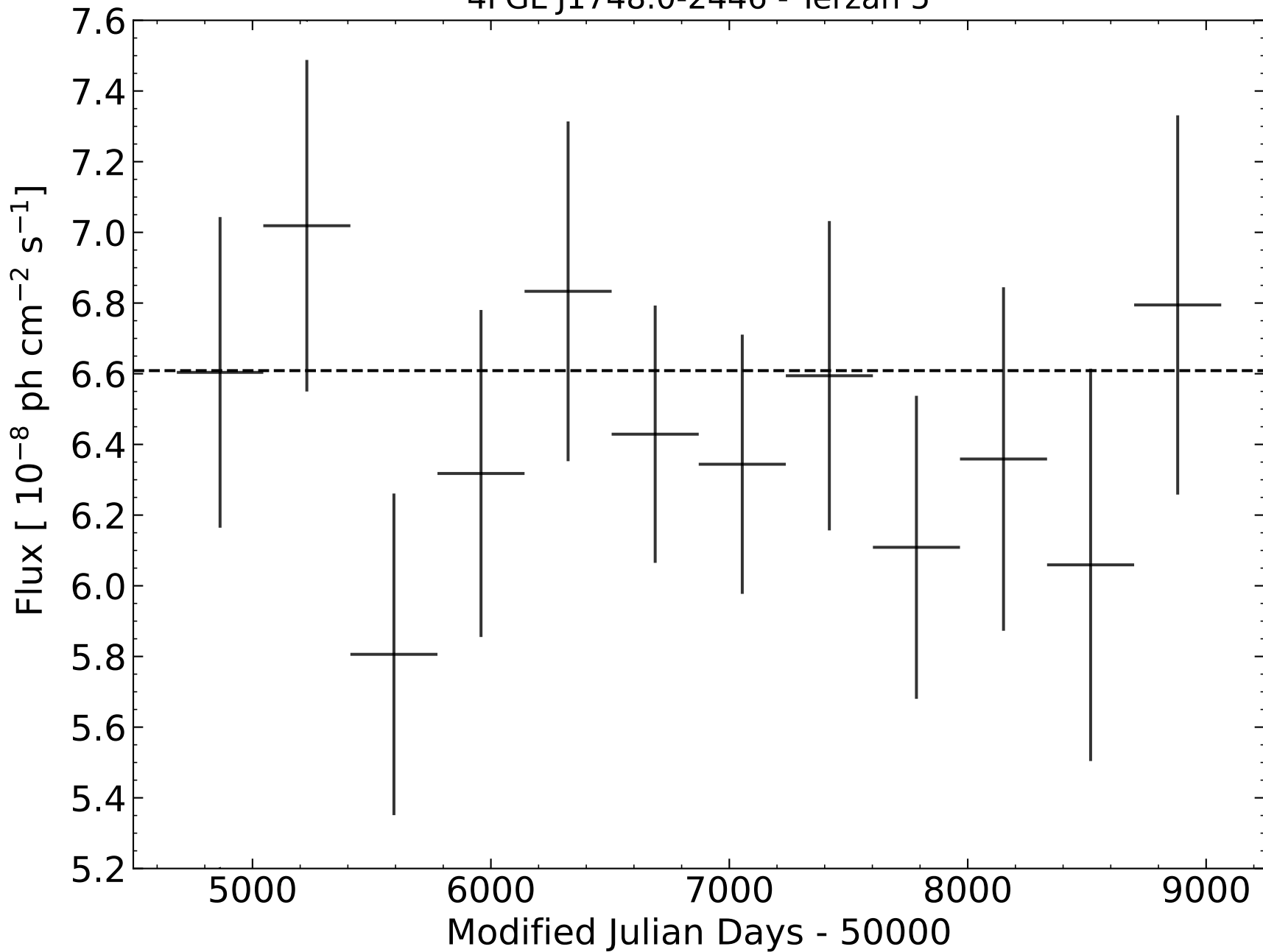
4FGL J1748.0-2446 - Terzan 5
