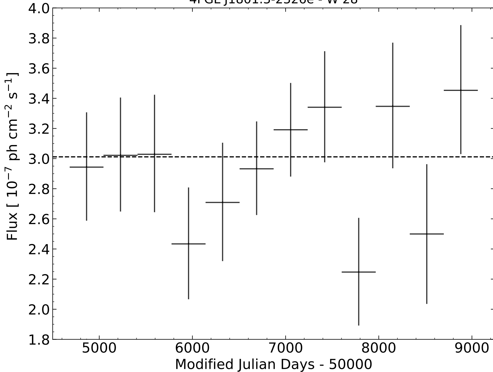
4FGL J1801.3-2326e - W 28
