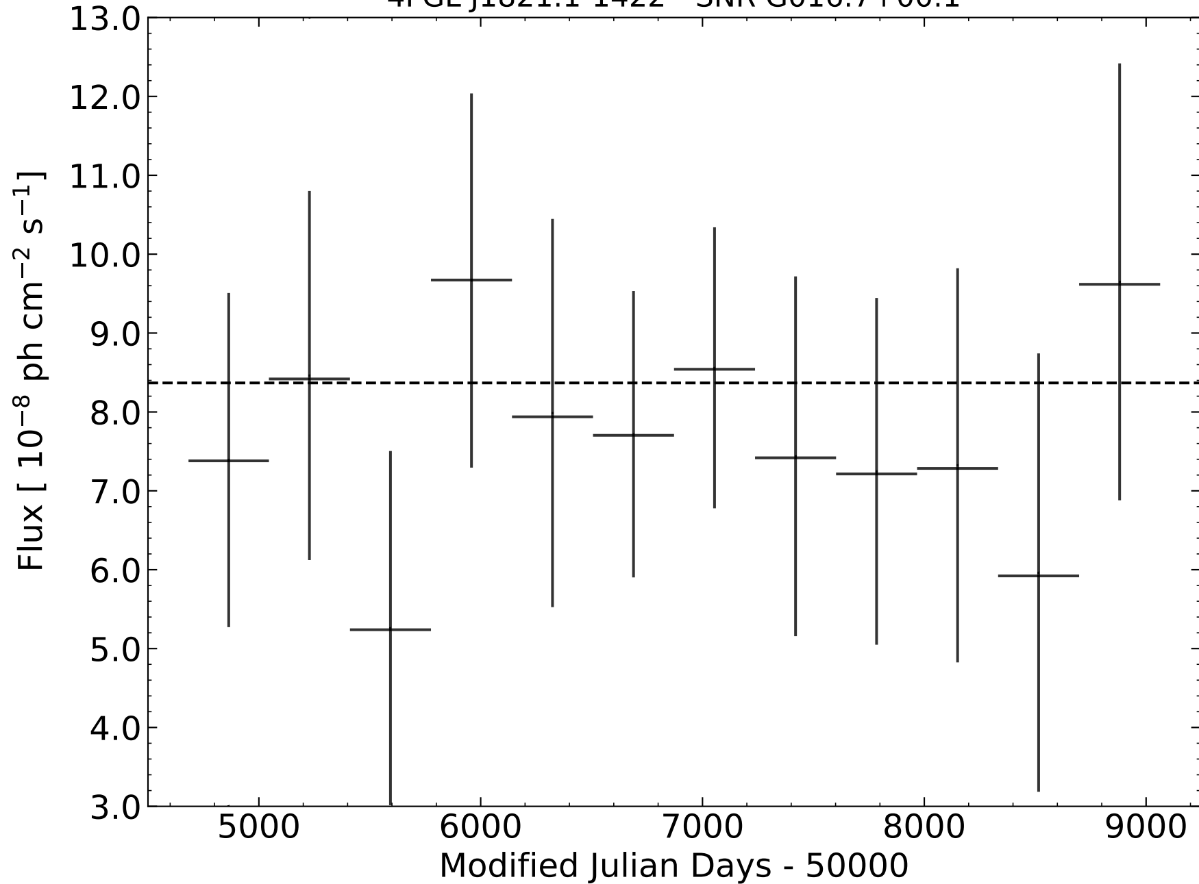
4FGL J1821.1-1422 - SNR G016.7+00.1
