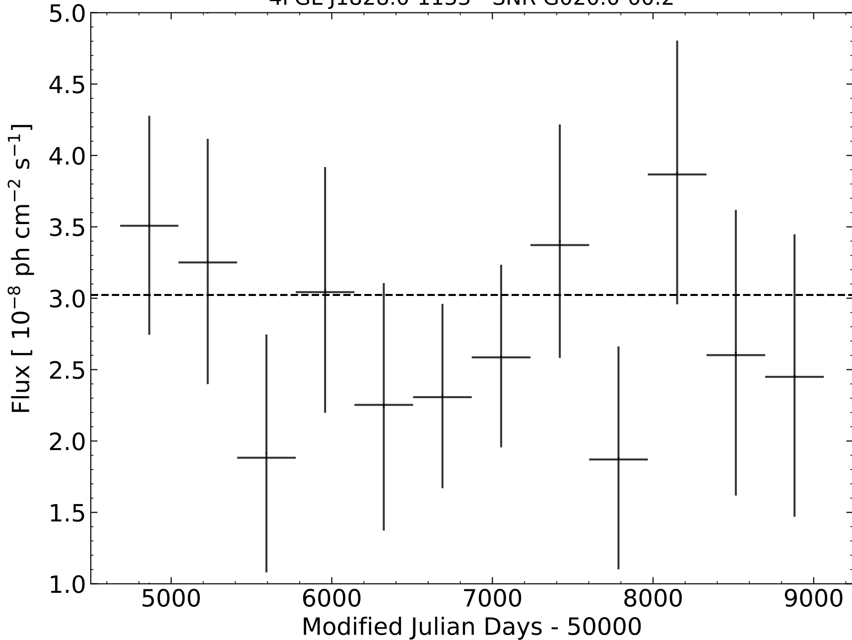
4FGL J1828.0-1133 - SNR G020.0-00.2
