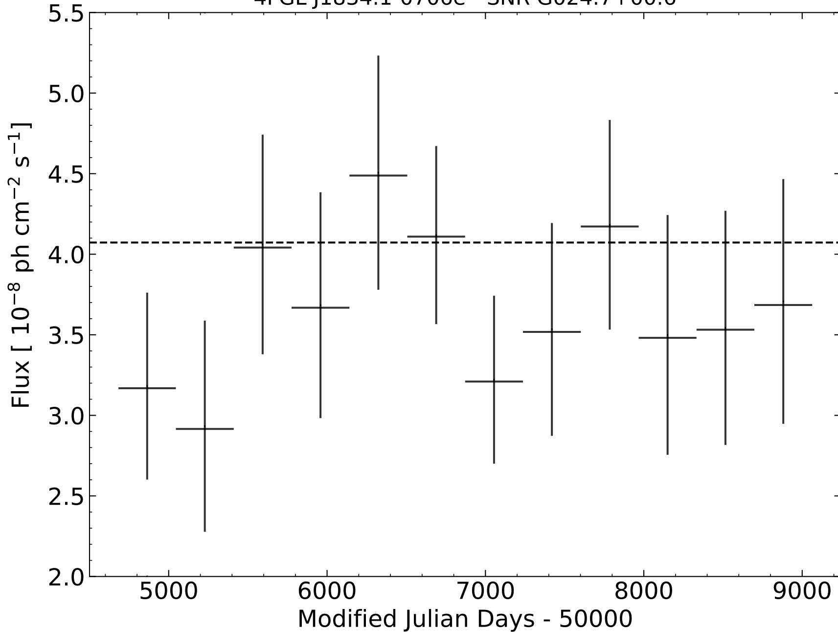
4FGL J1834.1-0706e - SNR G024.7+00.6
