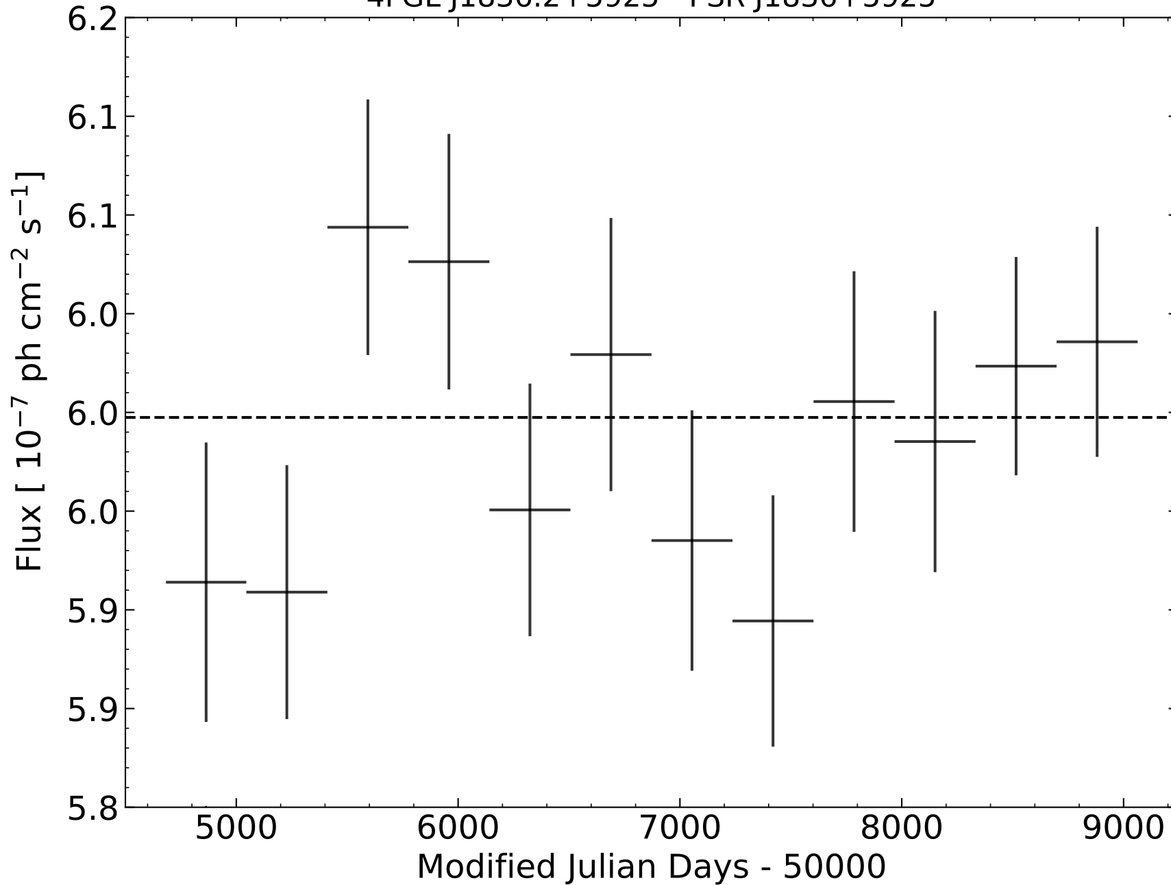
4FGL J1836.2+5925 - PSR J1836+5925
