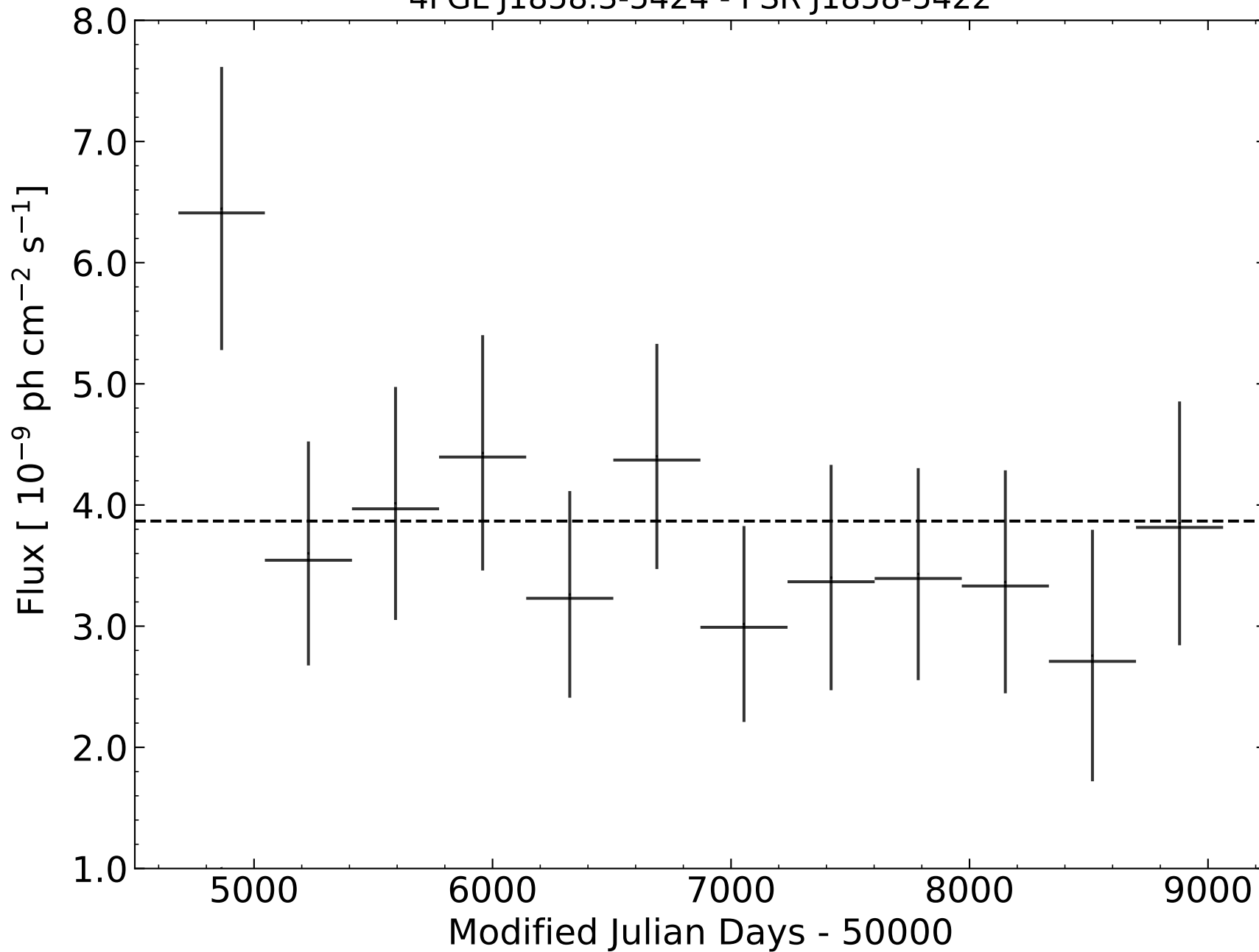
4FGL J1858.3-5424 - PSR J1858-5422
