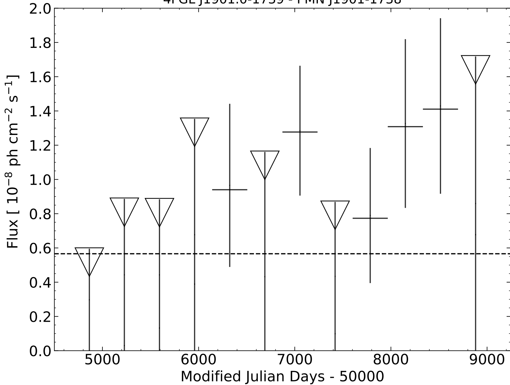
4FGL J1901.0-1739 - PMN J1901-1738
