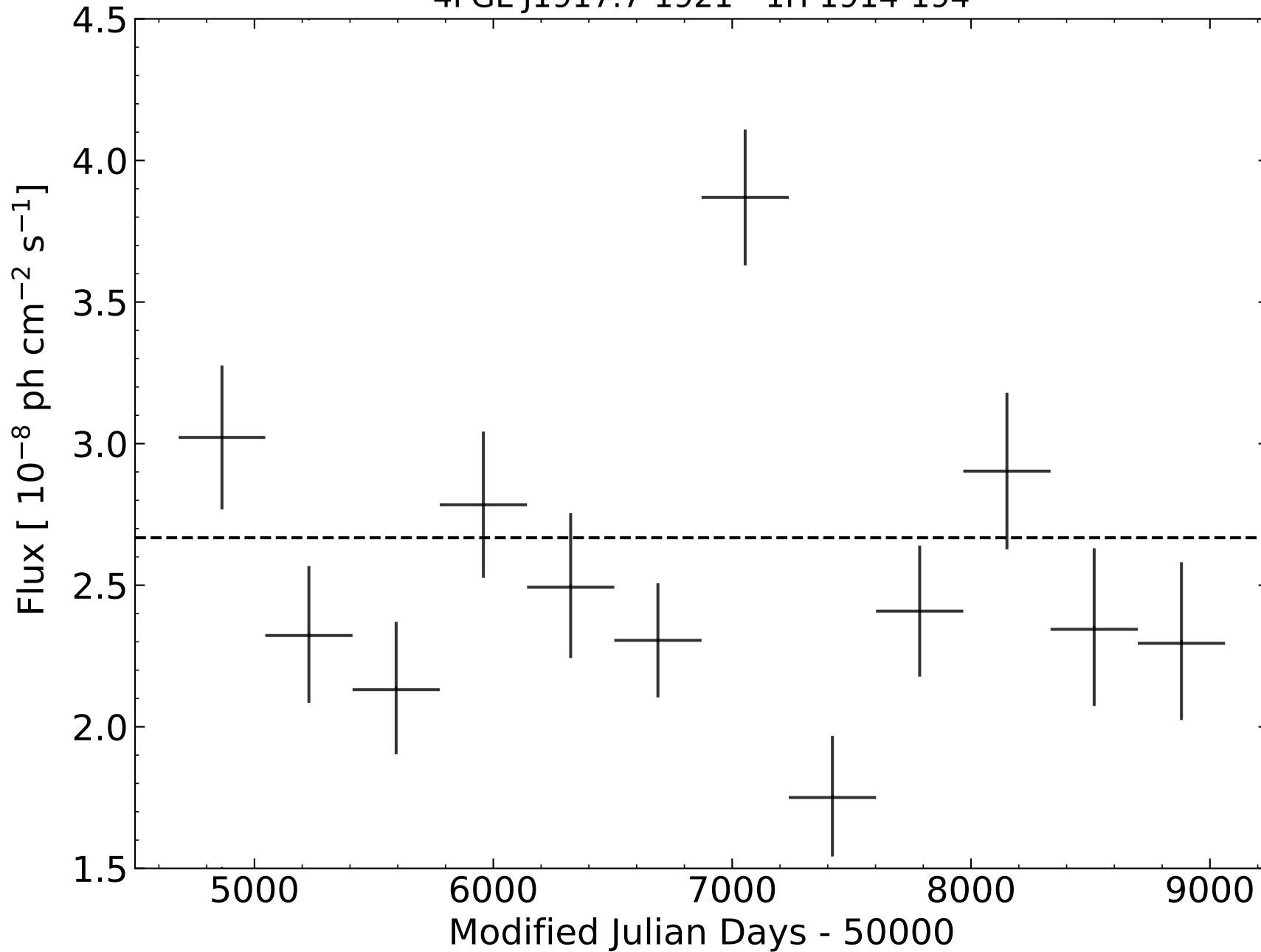
4FGL J1917.7-1921 - 1H 1914-194
