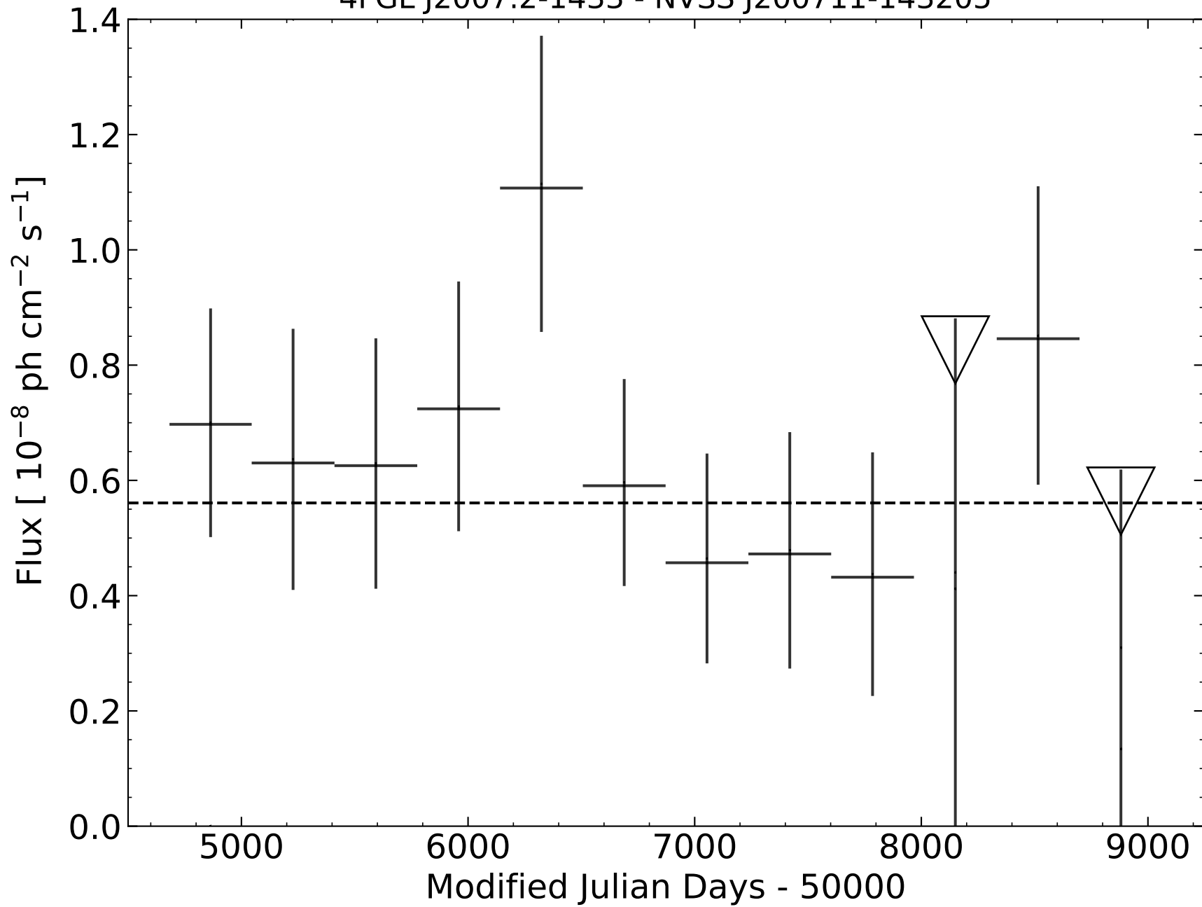
4FGL J2007.2-1433 - NVSS J200711-143205
