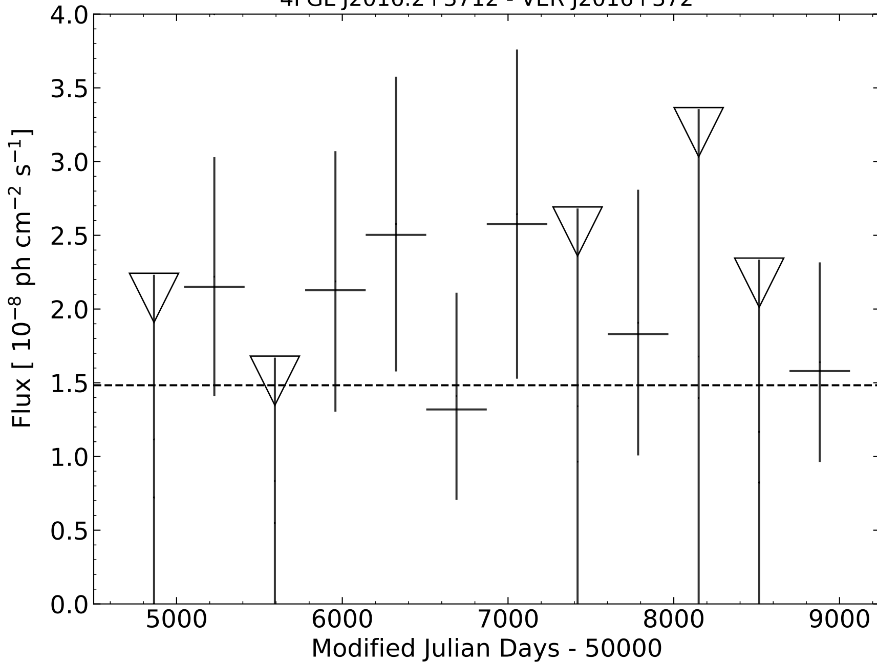
4FGL J2016.2+3712 - VER J2016+372
