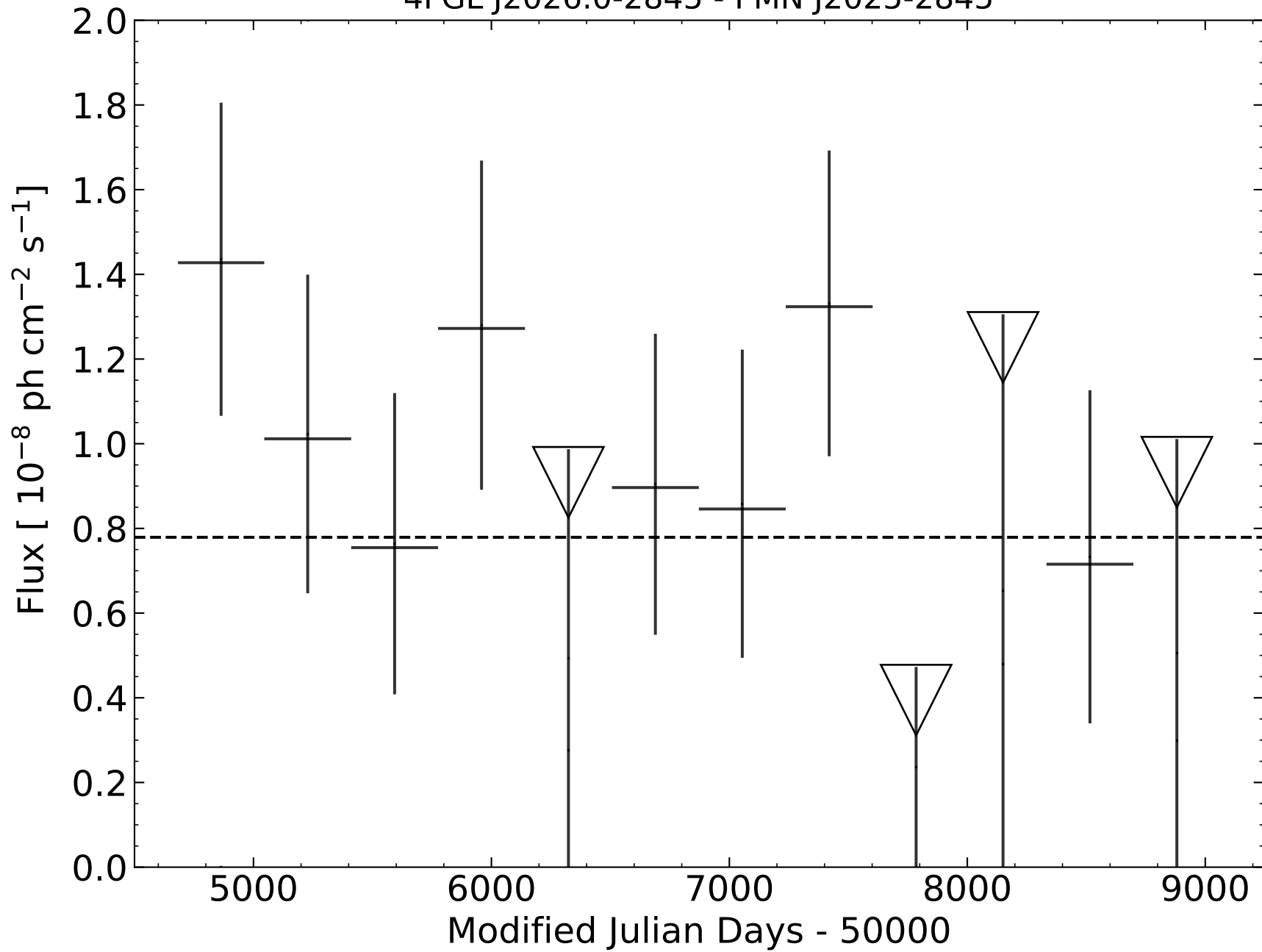
4FGL J2026.0-2845 - PMN J2025-2845
