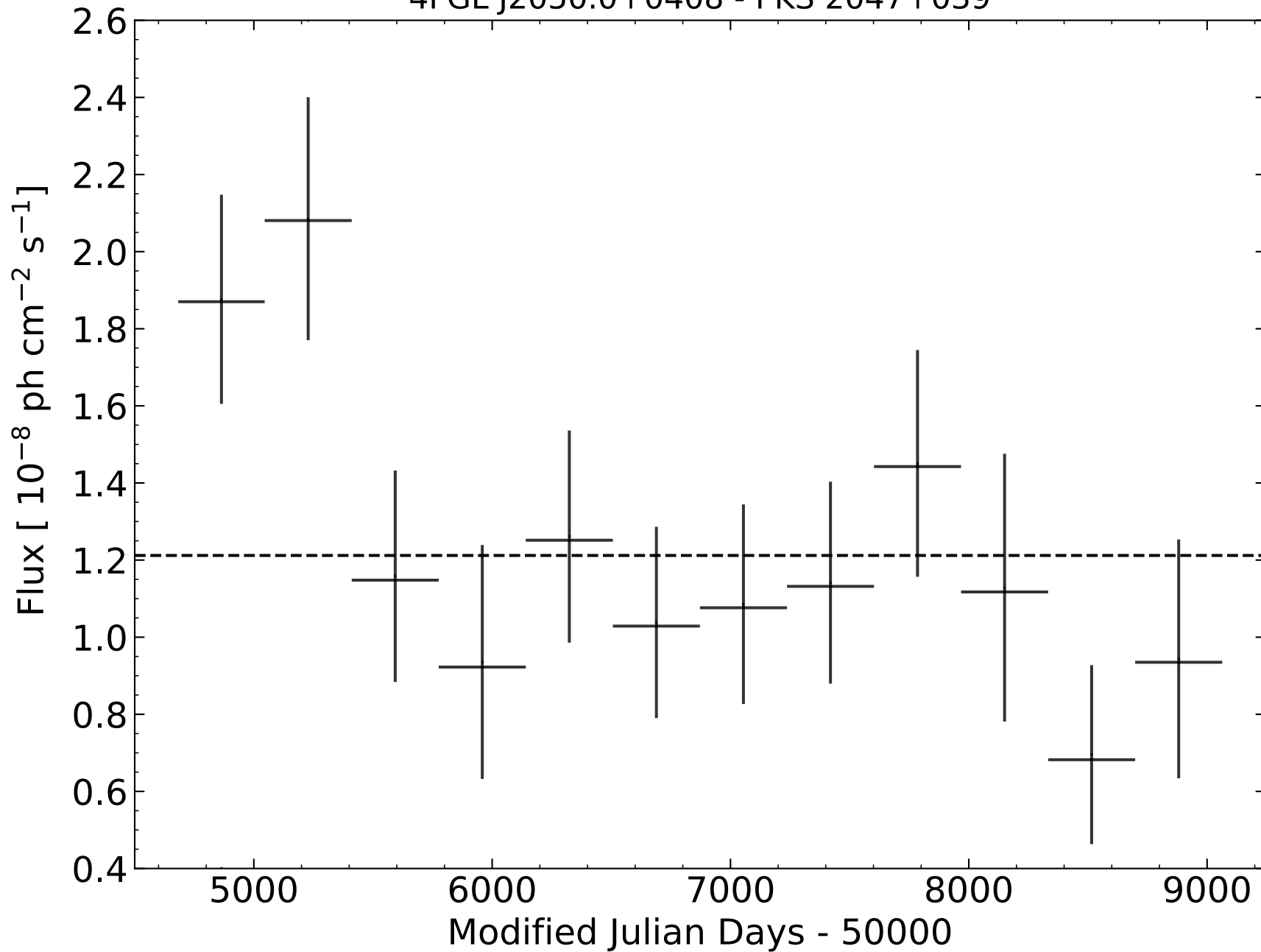
4FGL J2050.0+0408 - PKS 2047+039
