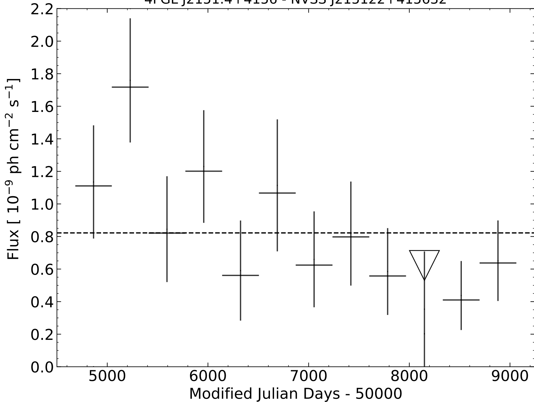
4FGL J2151.4+4156 - NVSS J215122+415632
