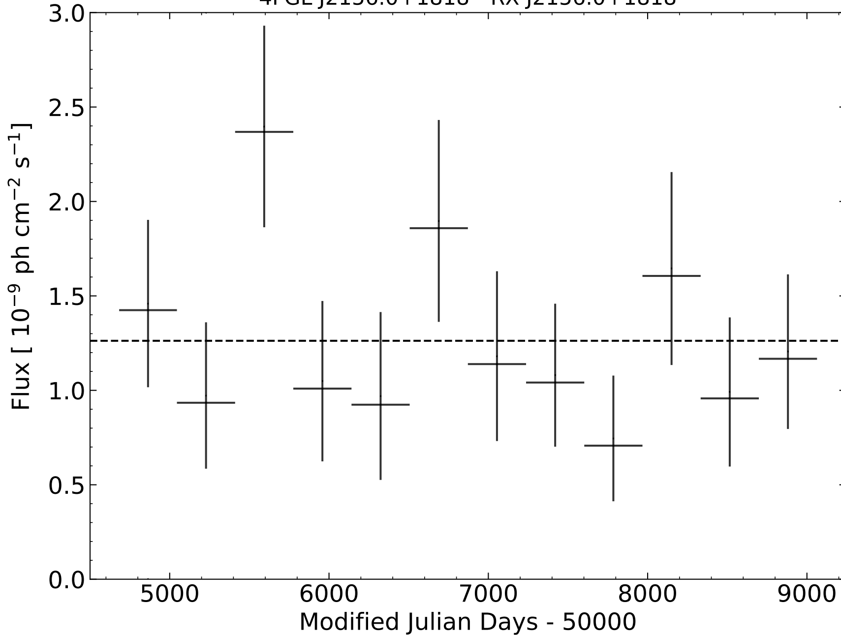
4FGL J2156.0+1818 - RX J2156.0+1818
