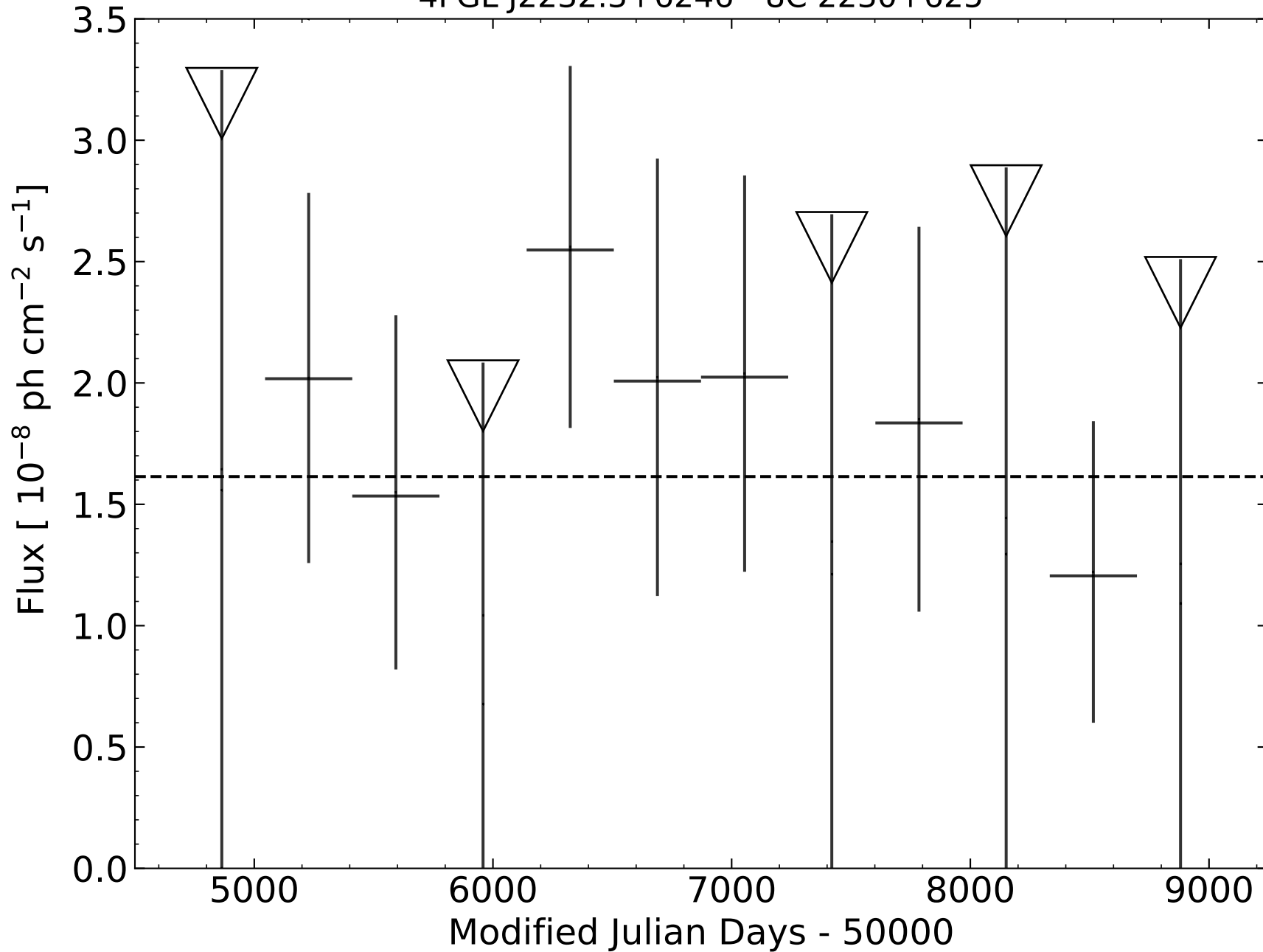
4FGL J2232.3+6246 - 8C 2230+625
