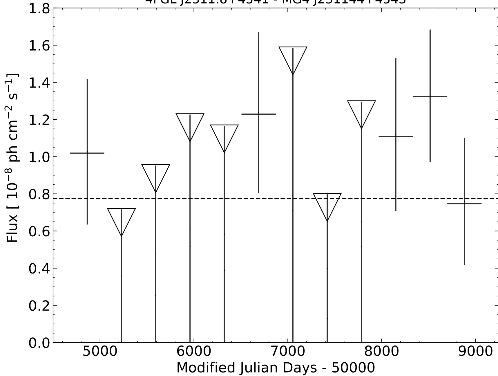
4FGL J2311.8+4541 - MG4 J231144+4543
