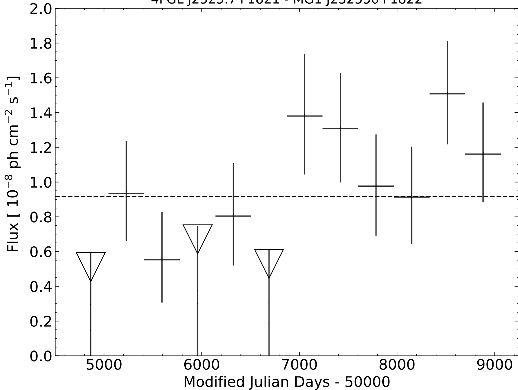
4FGL J2325.7+1821 - MG1 J232550+1822
