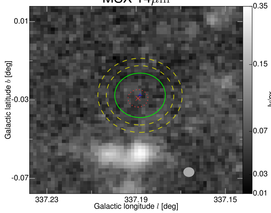
MSX 14\mu\text{m}
