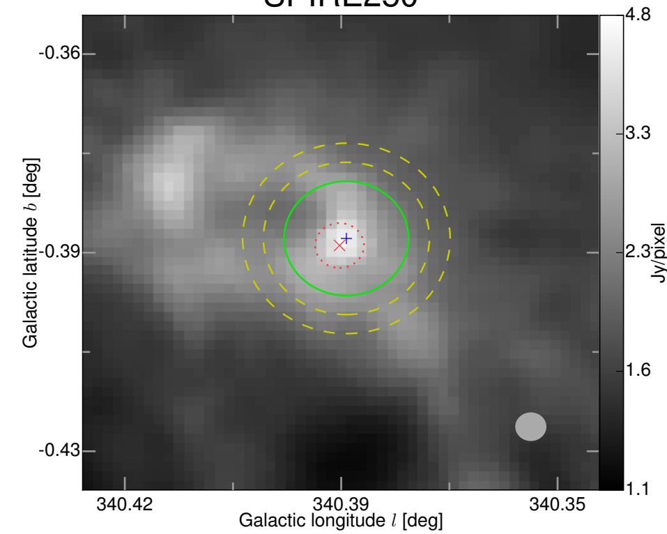
SPIRE250
