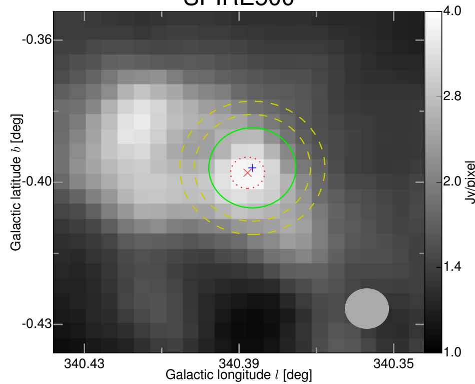
SPIRE500
