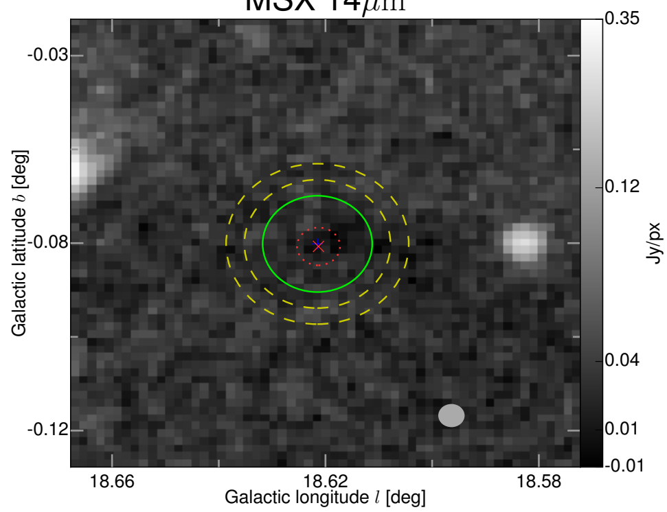
MSX 14\mu\text{m}
