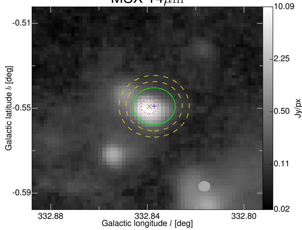
MSX 14 \mu\text{m}
