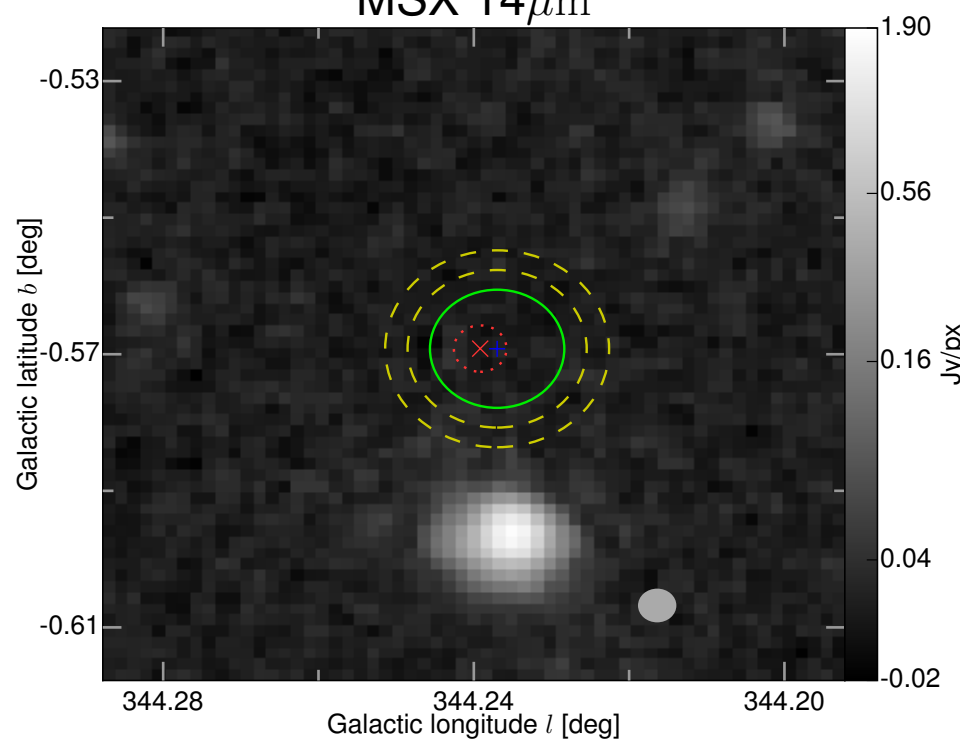
MSX 14 \mu\text{m}
