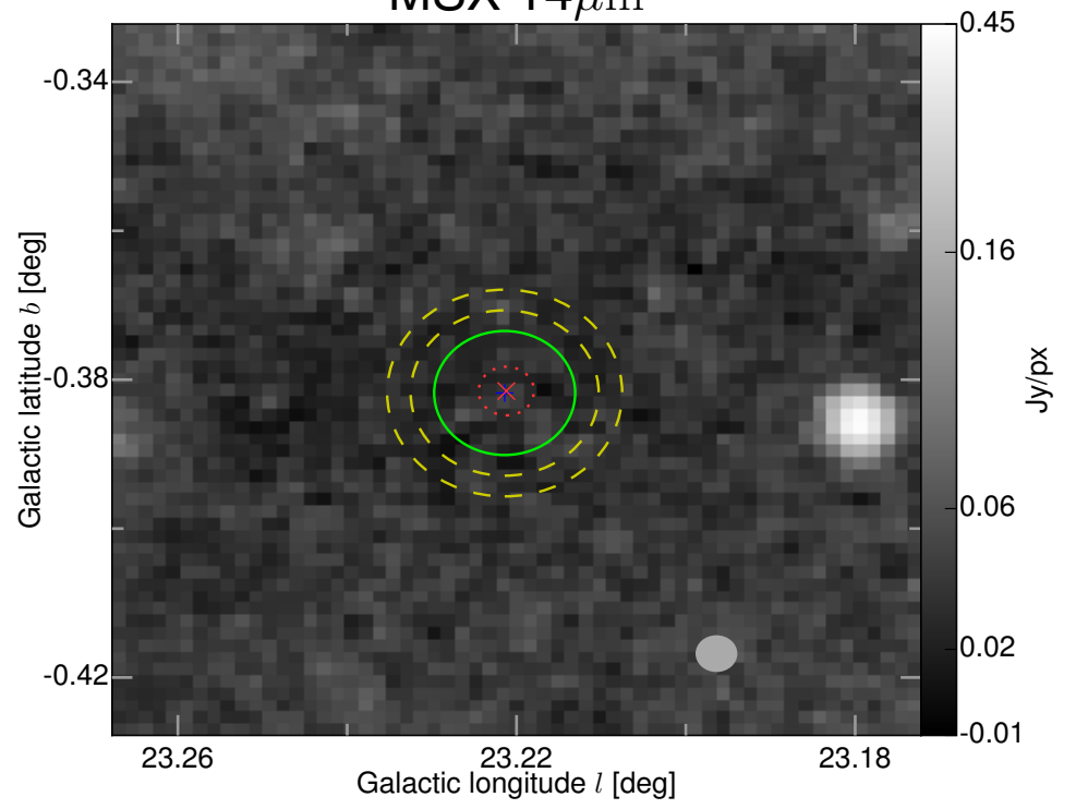
MSX 14 \mu\text{m}
