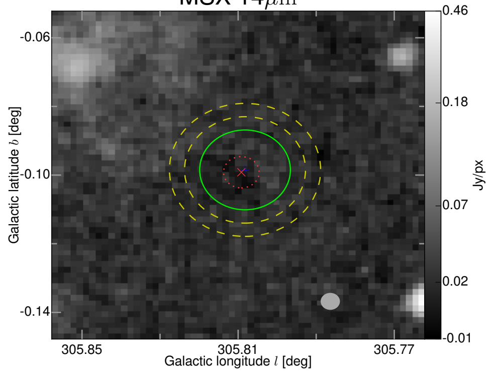
MSX 14 \mu\text{m}
