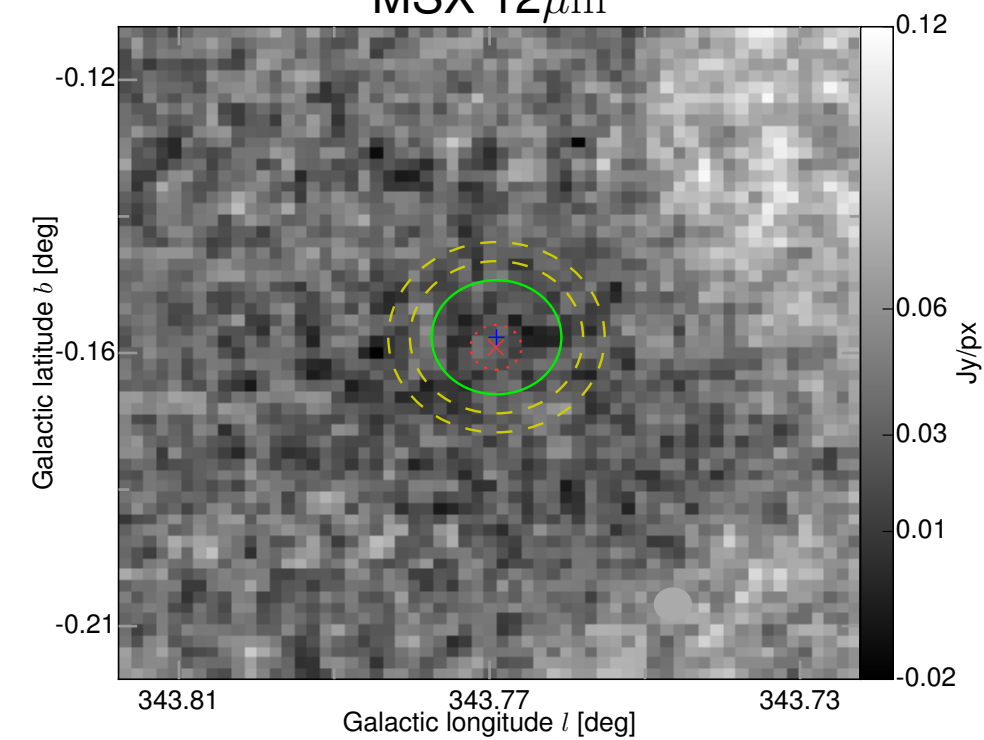
MSX 12\mu\text{m}
