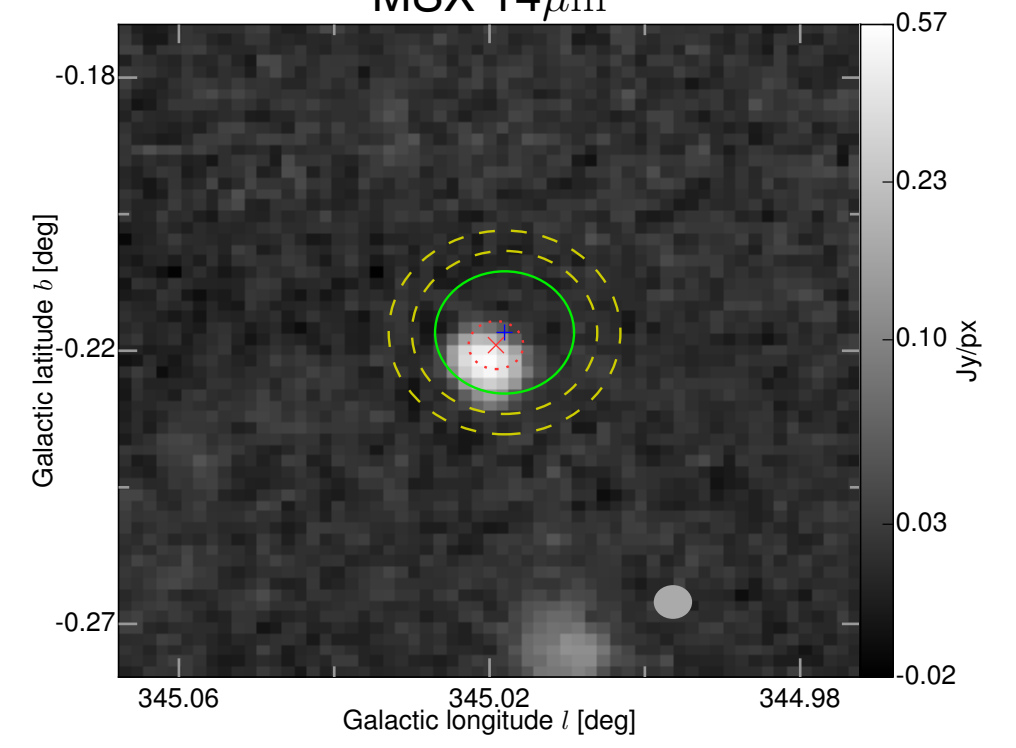
MSX 14 \mu m
