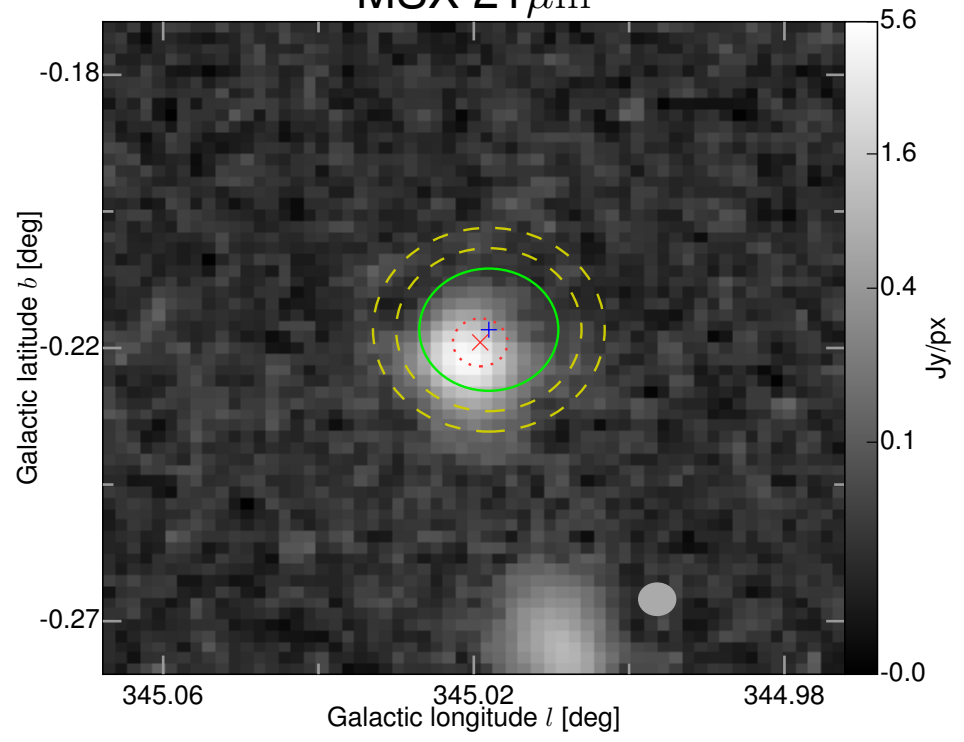
MSX 21 \mu m
