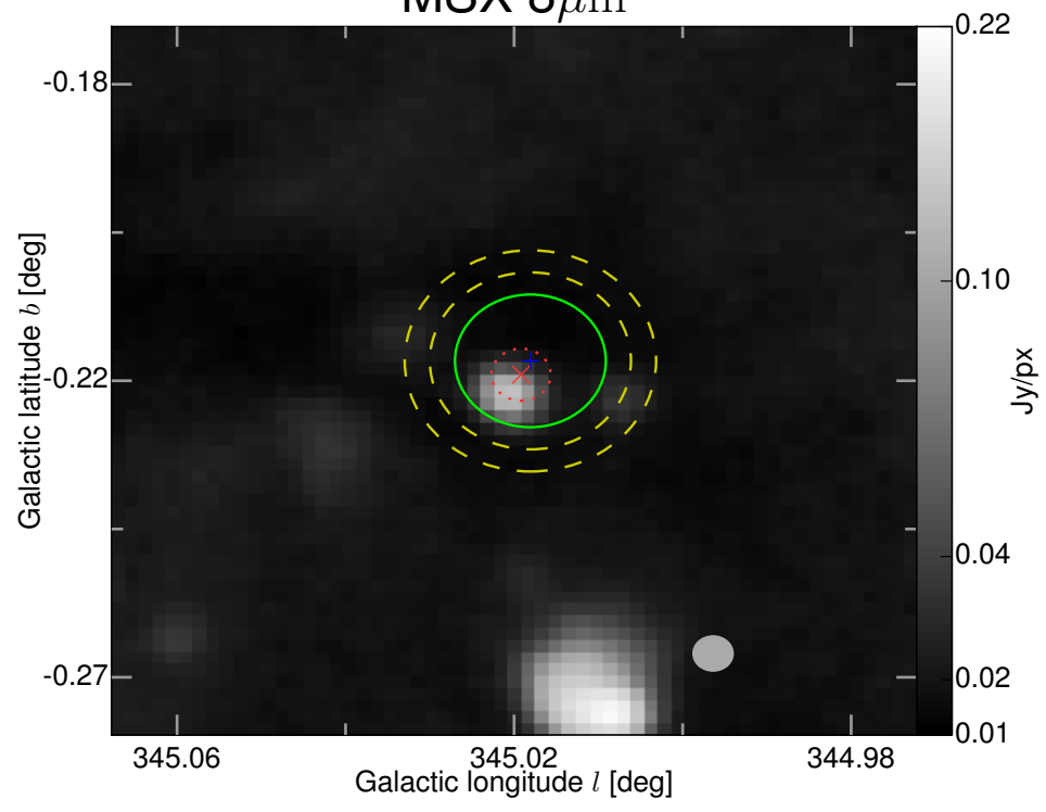
MSX 8 \mu m
