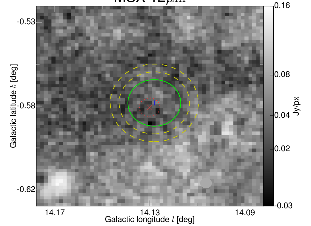
MSX 12\mu\text{m}
