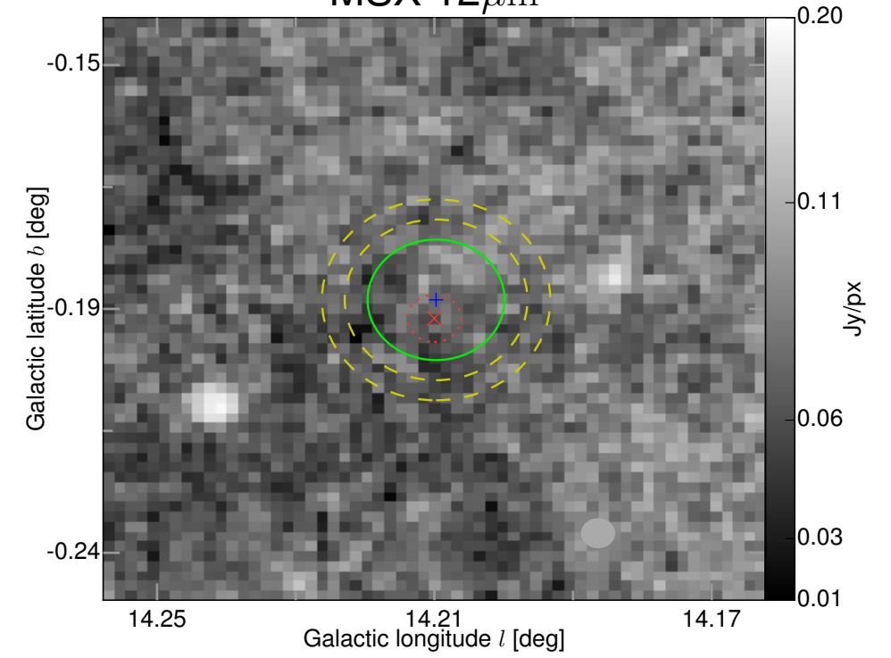
MSX 12\mu\text{m}
