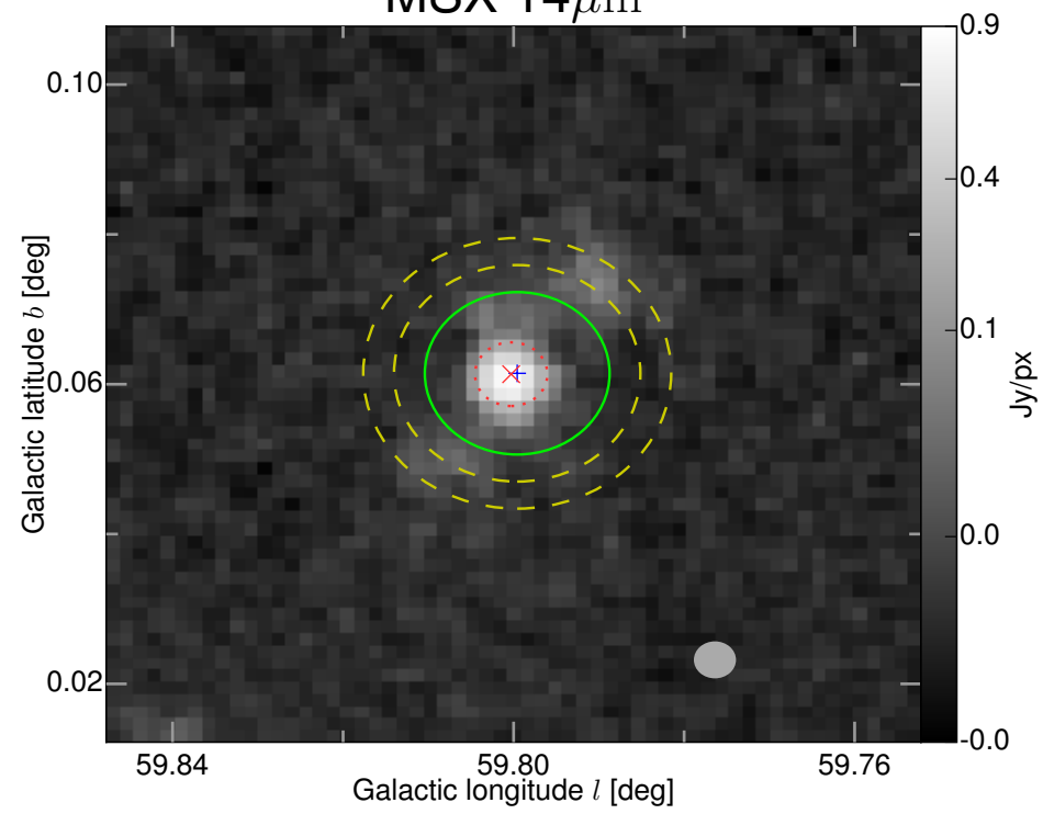
MSX 14\mu\text{m}
