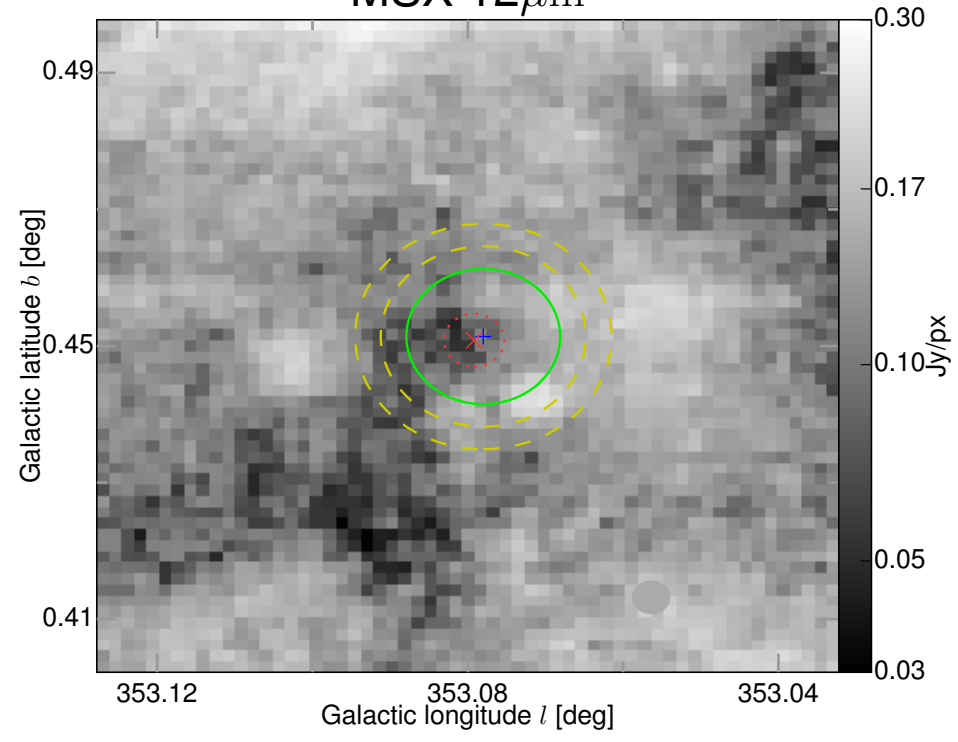
MSX 12 \mu m
