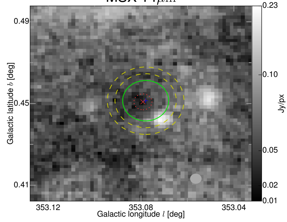
MSX 14 \mu m
