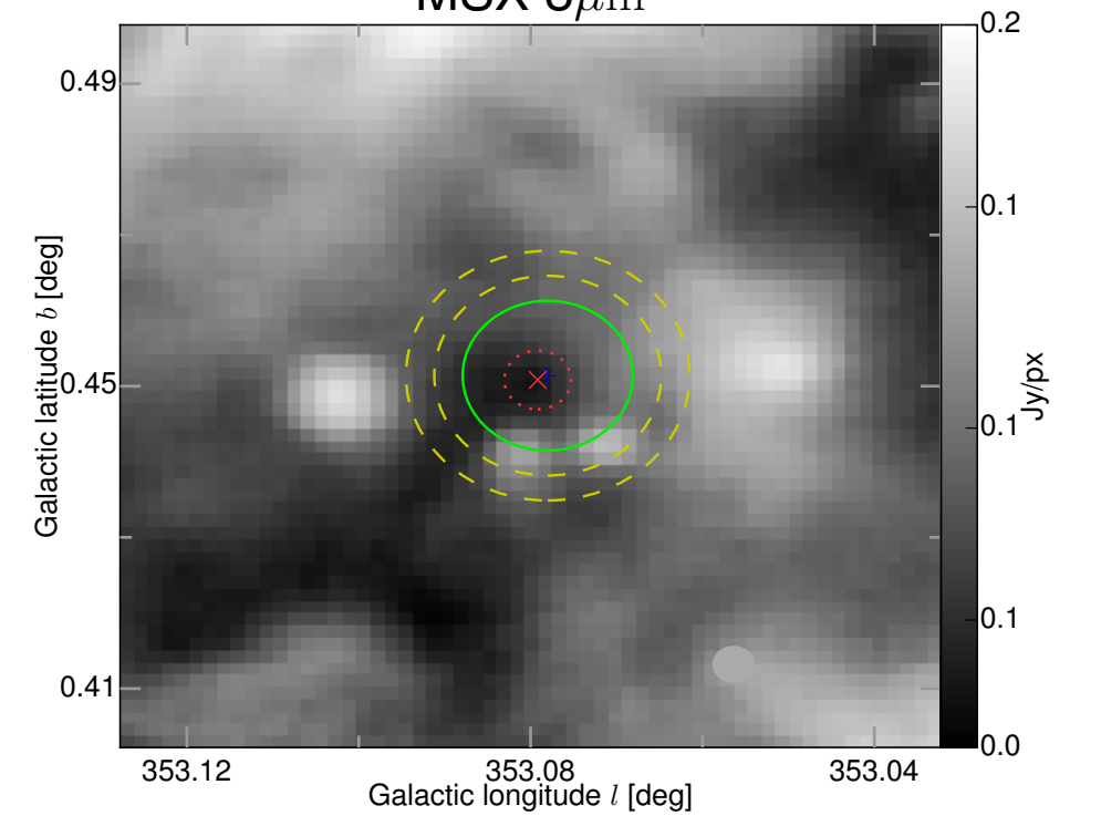
MSX 8 \mu m
