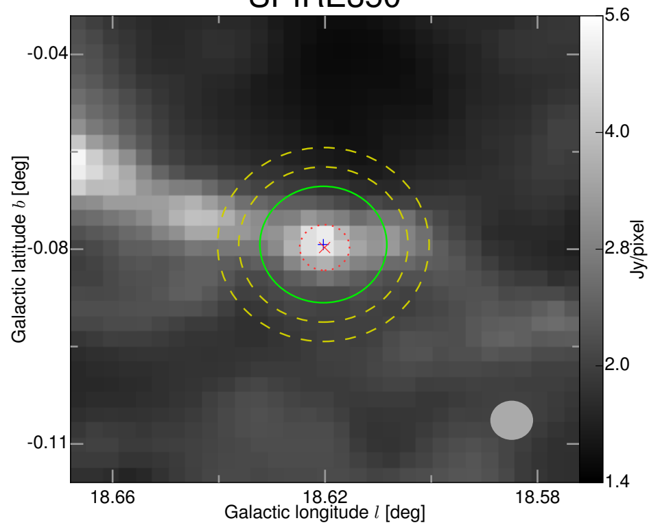
SPIRE350
