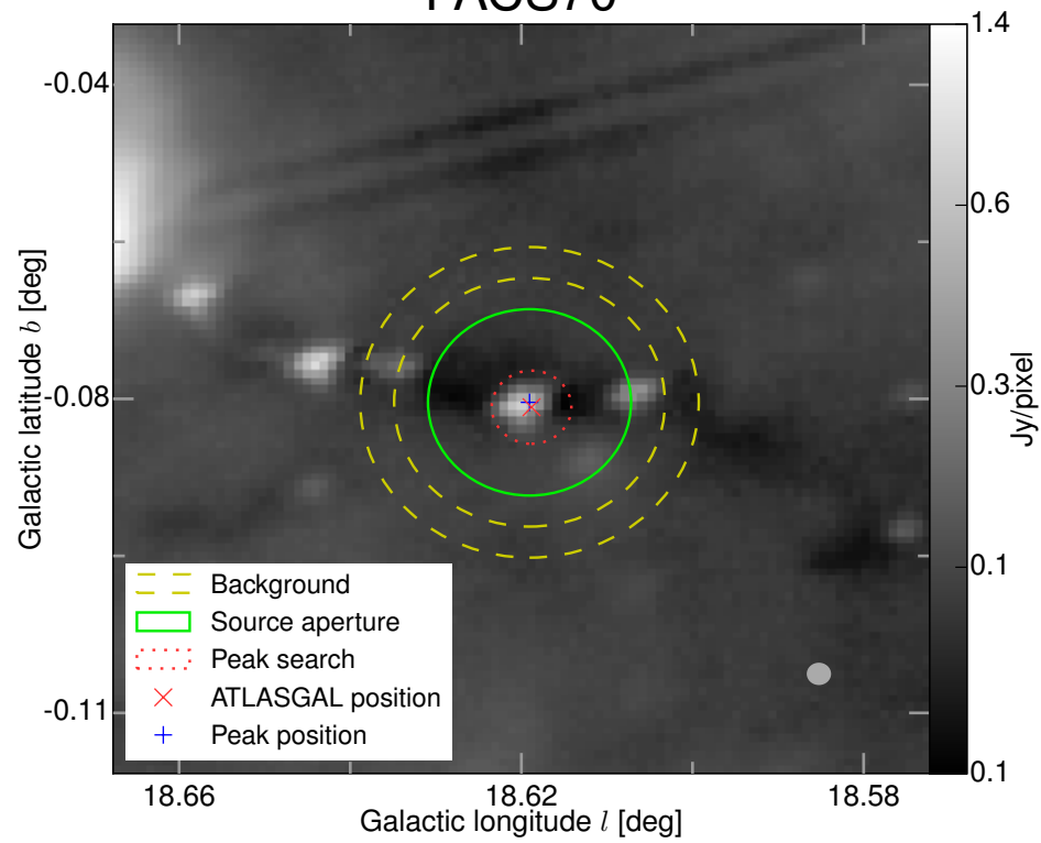
PACS70
