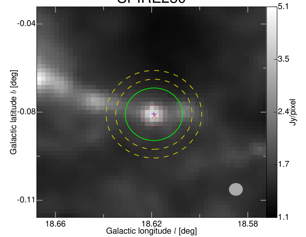
SPIRE250
