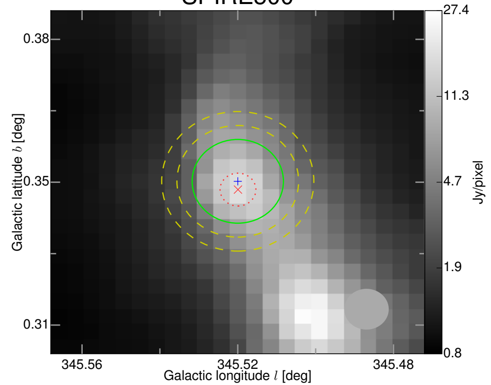
SPIRE500
