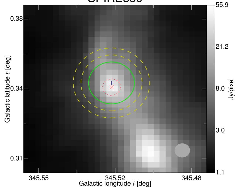
SPIRE350
