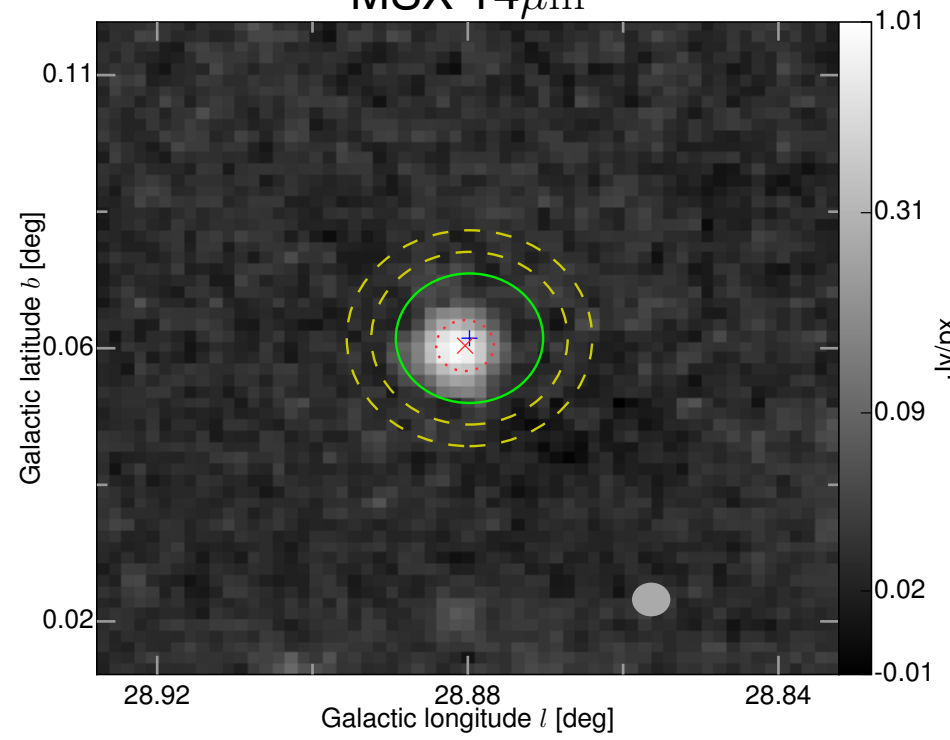
MSX 14\mu\text{m}
