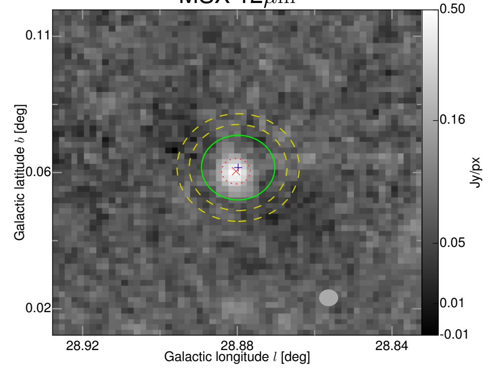
MSX 12\mu\text{m}
