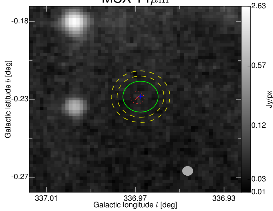
MSX 14 \mu\text{m}
