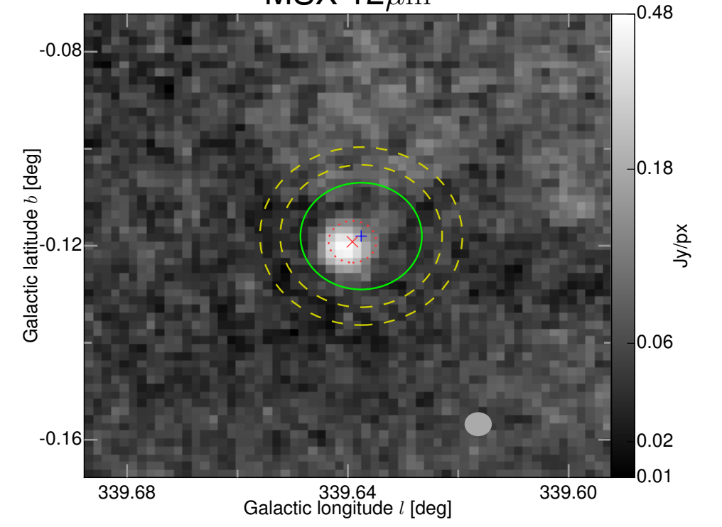
MSX 12\mu\text{m}
