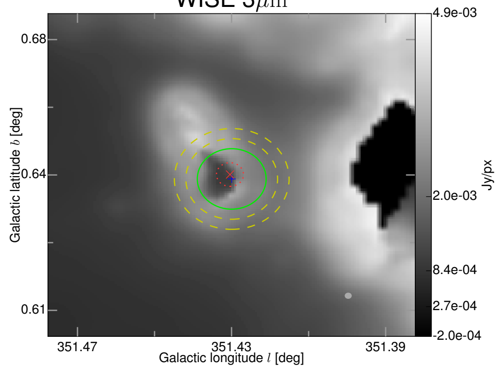
WISE 3\mu\text{m}
